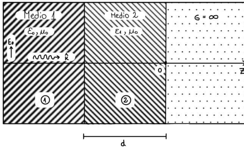
Figura 3: Placa dieléctrica de dos medios.
