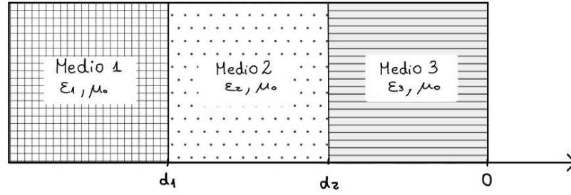
Figura 2: Tres medios con el último adosado a un plano perfectamente conductor.
