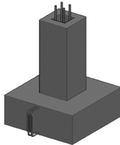
VISTA ISOMETRICA FUNDACION 002
