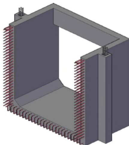
VISTA ISOMETRICA FRONTAL
