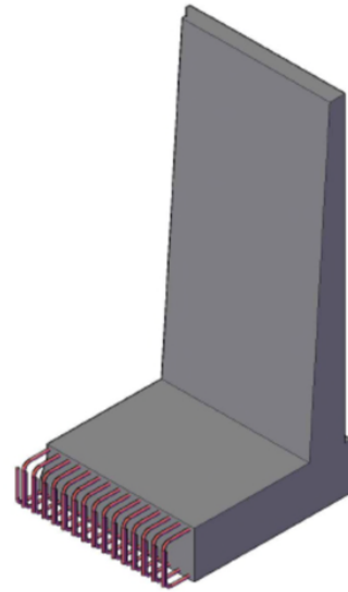
VISTA ISOMETRICA MURO
