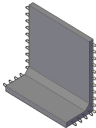
VISTA ISOMETRICA FUNDACION
