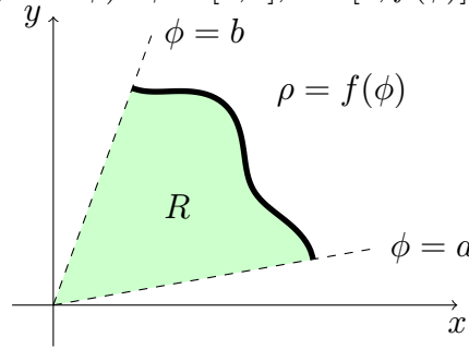
Figura 8: Región en coordenadas polares.
