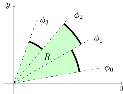
Figura 9: Región en coordenadas polares para f escalonada.
