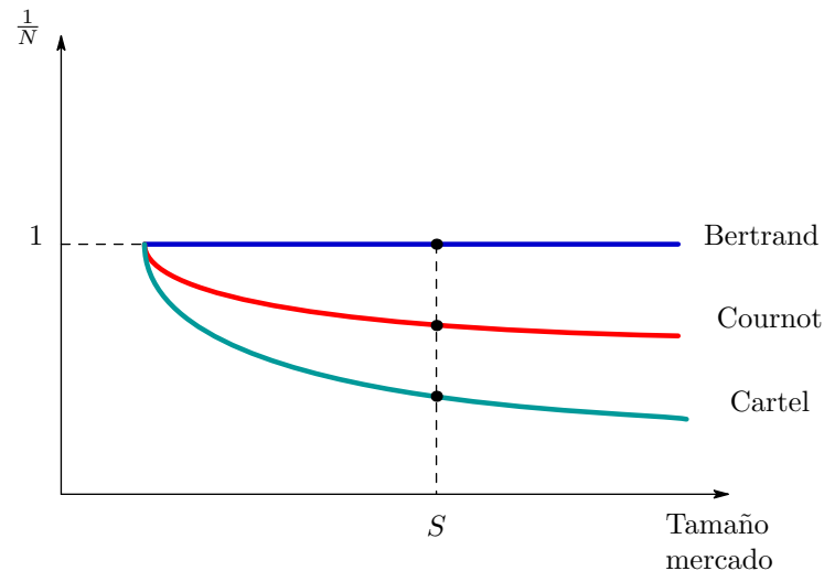
Figura 12.16: Concentración y tamaño de mercado
