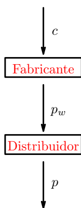
Figura 7.6: Doble marginalización
