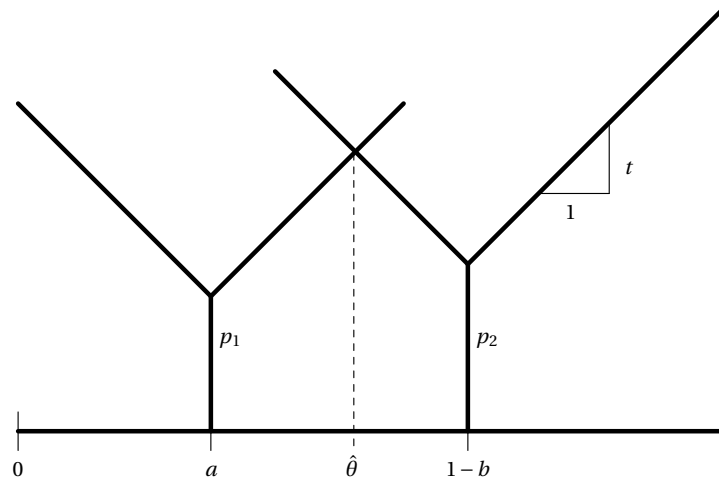
Figura 10.10: Precios ajustados por localización, con costos lineales.
