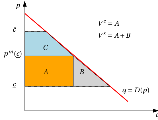
Figura 14.7: Incentivos a la innovación bajo competencia V^c y planificador social V^s
