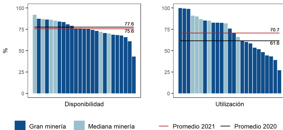
Figura 13: Indicadores de productividad del activo carguío en mina rajo, año 2021.
