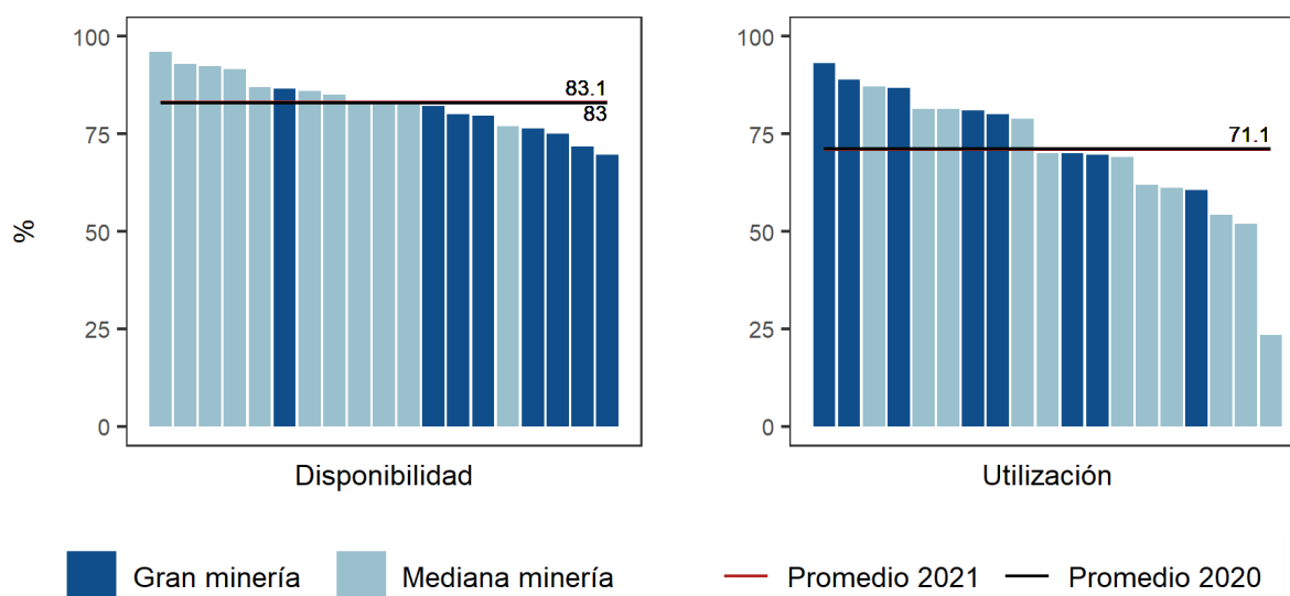
Figura 18: Indicadores de productividad del área seca en planta hidrometalúrgica, año 2021.
