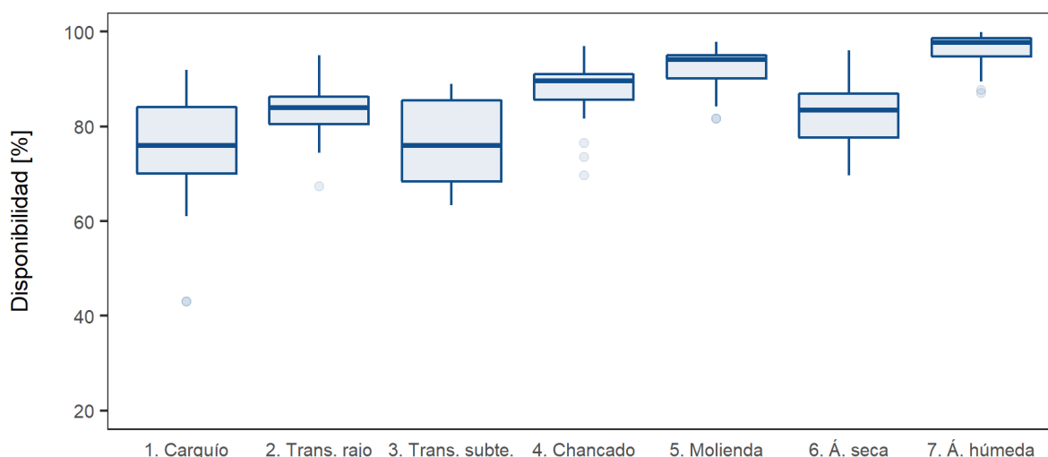
Figura 20: Resumen de indicadores de disponibilidad, año 2021.
