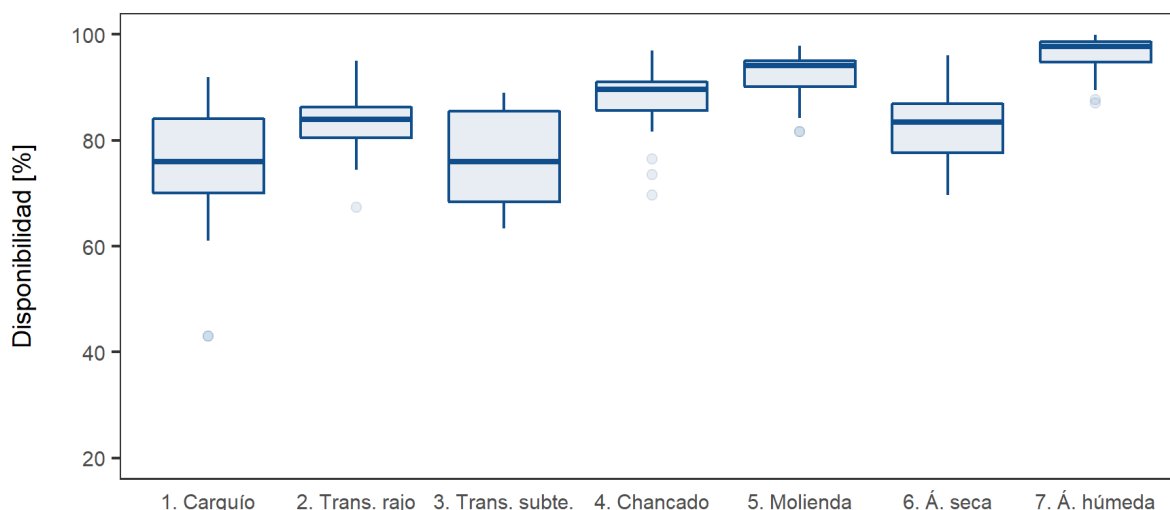
Figura 2: Resumen de indicadores de disponibilidad, año 2021.
