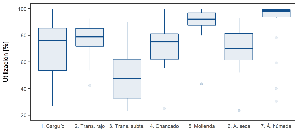
Figura 3: Resumen de indicadores de utilización, año 2021.
