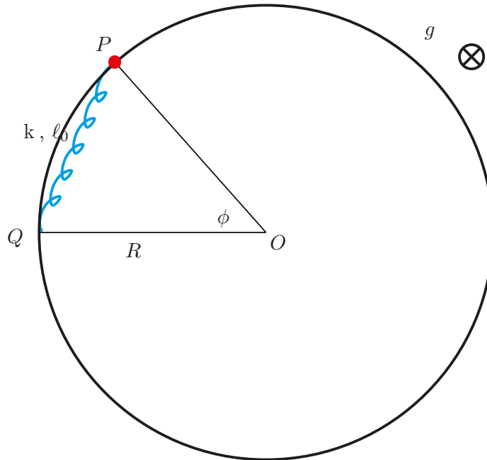
Figure 1: Partícula P en cilindro vertical.
