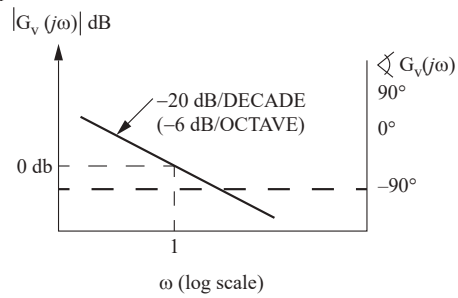
(d) (1 + j\omega/\omega_c)
