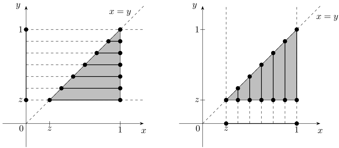
Figura 1: Región de integración R
