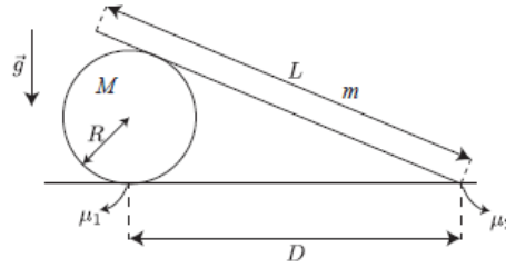
Figura 6.3: Barra con pivote.
