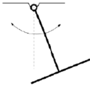
Figura 7.5: Péndulo físico.
