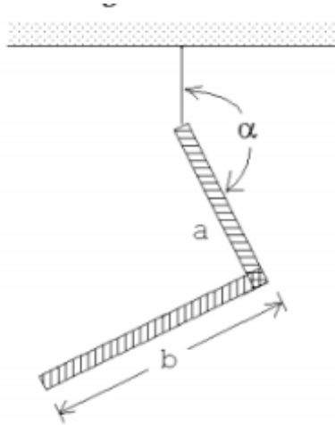
Figura 6.1: Montaje en forma de L colgando desde un extremo por un hilo.
