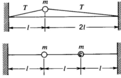
Figura 8.1: Oscilaciones transversales acopladas
