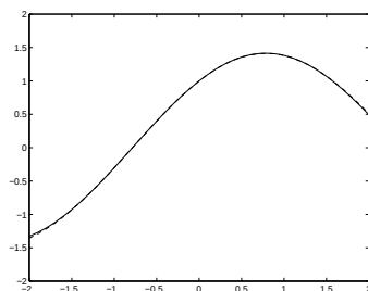
T_f^6(x)
