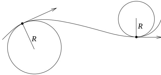
vector tangente y curvatura.
