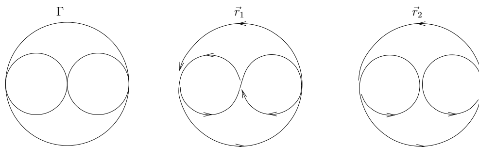
Parametrizaciones no equivalentes para la misma curva \Gamma
