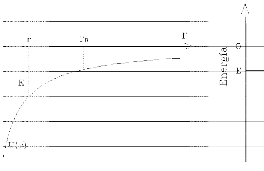
Figura 11.8 : Potencial efectivo para \ell = 0 .
