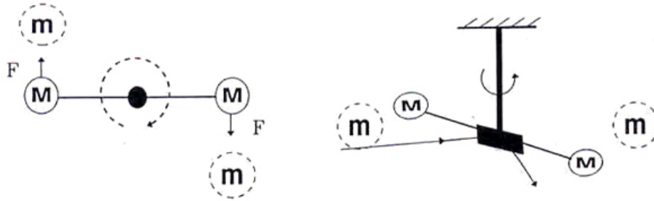
Figura XV.3: La Figura muestra el diseño del péndulo de torsión empleado por Cavendish para medir la constante de gravitación G . El espejo refleja un haz de luz incidente, que permite detectar pequeñas rotaciones de la barra.
