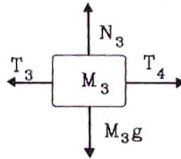
Figura VI.12: Diagrama de cuerpo libre de la masa que representa a la cuerda. Como no existe movimiento en la dirección vertical, su aceleración en esa dirección es nula.
