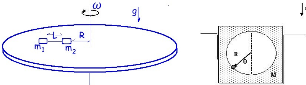
Figura VI.30: DCL para dos poleas y tres masas. La reacción sobre el piso debido al movimiento circular.
