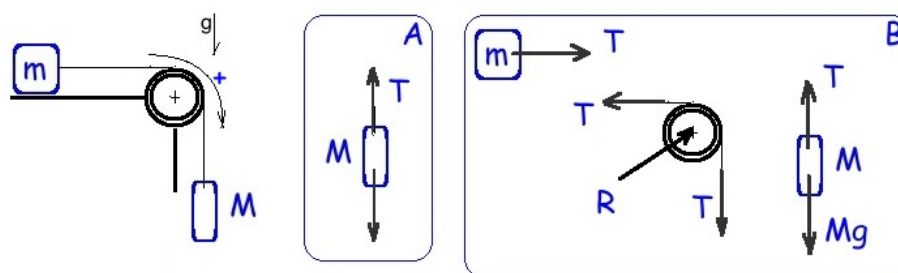
Figura VI.5: La fuerza \mathbf{R} indicada en la figura B representa la reacción en el eje de la polea (supuesta sin masa o cuya masa es despreciable con respecto a la tensión que actúa en la cuerda). Si las tensiones son perpendiculares entre sí, la reacción apunta en 45^\circ .
