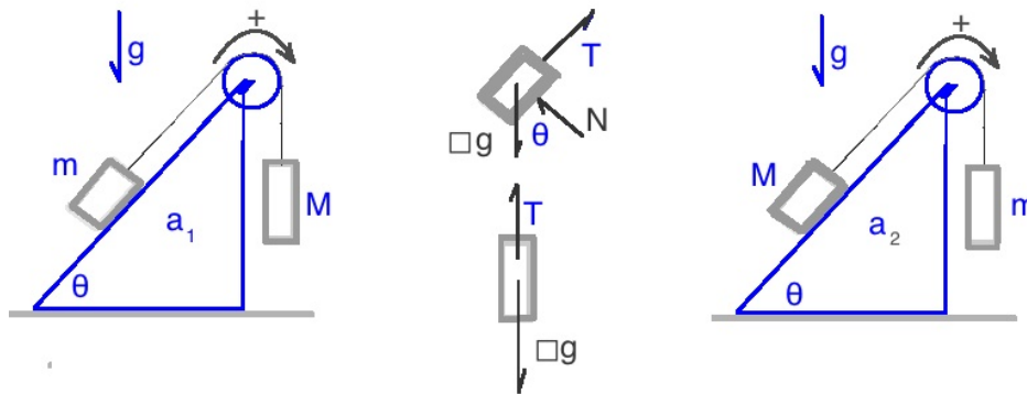
Figura VI.31: Se muestran las dos configuraciones definidas y los diagramas de cuerpo libre de las masas m y M . En los cuadrados incluidos al lado de g , se debe incluir la masa relevante al caso 1 o al caso 2.
