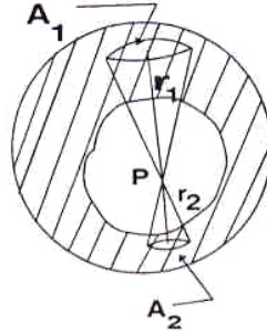
Figura XV.6: En la Figura se indican los conos geométricos utilizados en la demostración del Teorema I. Se supone que son infinitesimales, de manera que las aproximaciones tengan un error despreciable.
