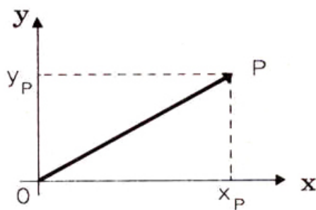
Figura V.1: La flecha \overrightarrow{OP} indica que el objeto se comporta como un vector. Las componentes de este vector, son las proyecciones del vector sobre el eje x , denominado abcisa y el eje y , la ordenada . Las coordenadas del punto P se escriben como un par ordenado de números reales, (x_P, y_P) . El primer número, x_P , se obtiene trazando una paralela al eje y a través del punto P .
