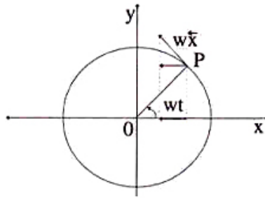
Figura IX.3: La velocidad se puede obtener geométicamente de la Figura. Es tangente a la circunferencia y su magnitud está dada por el producto del radio por la velocidad angular. La velocidad de la masa unida al extremo del resorte se obtiene proyectando w r sobre el eje x .
