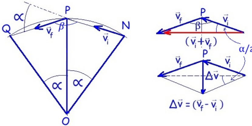
Figura V.51: Los resultados obtenidos a continuación se desprenden de las propiedades de los triángulos isósceles que emergen de la naturaleza del problema.
