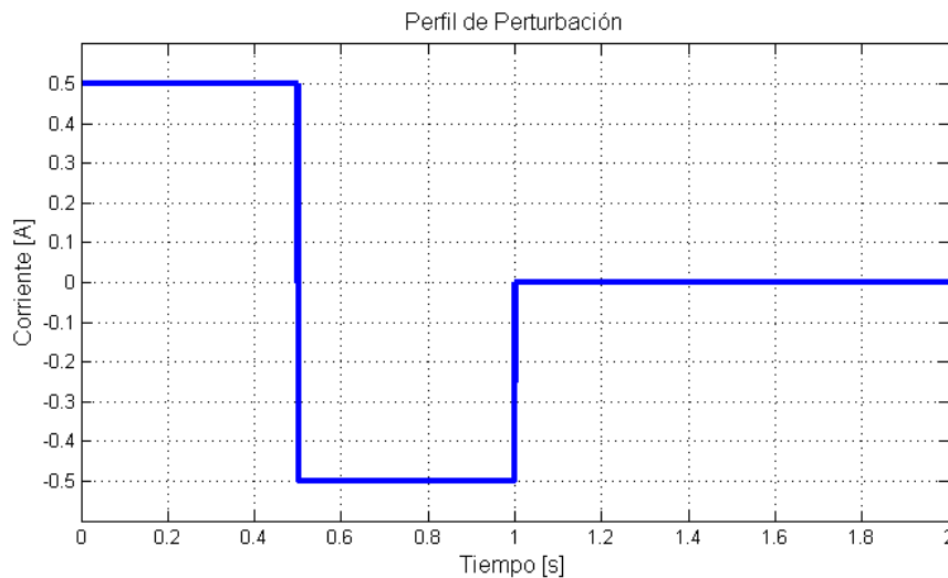
Figura 3: Perfil de perturbación para prueba de reducción de oscilaciones
