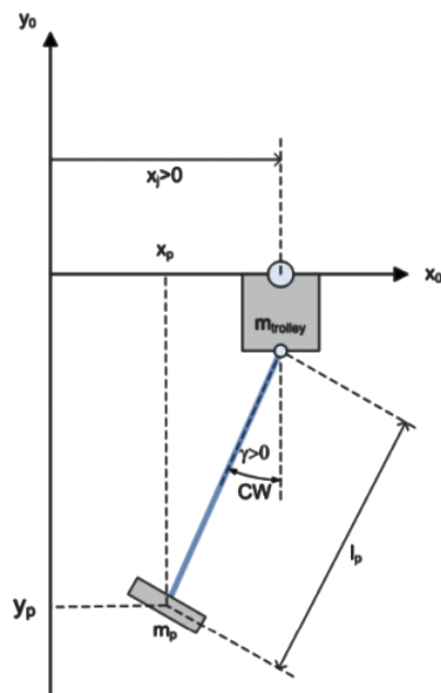
(b) Diagrama de Cuerpo Libre. Subsistema Brazo
