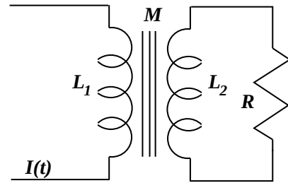
Figura 6.19: Un transformador cuyo secundario está conectado a una resistencia R .
