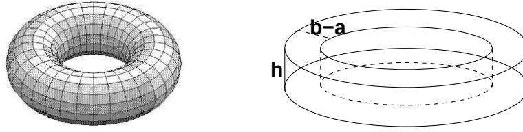
Figura 5.5: A la izquierda un núcleo toroidal de sección circular y a la derecha un núcleo toroidal de sección rectangular.
