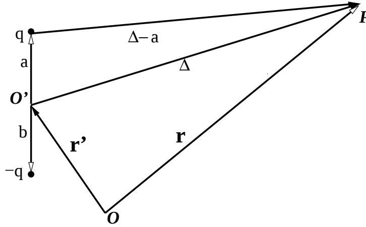
Figura 1.4: Dos cargas q y -q separadas por una distancia a + b crean un campo en P cuya aproximación dipolar (1.6.1) es de interés.
