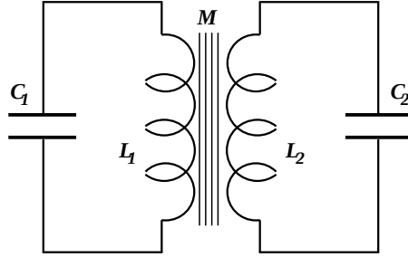
Figura 6.20: Dos circuitos LC con acoplamiento M .
