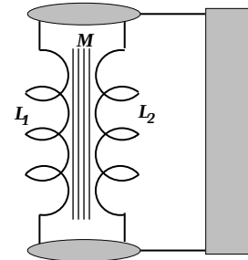
Figura 6.16: Un circuito genérico con dos inductancias L_1 y L_2 acopladas.
