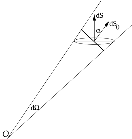
Figura 1.3: El elemento de superficie dS se relaciona al elemento de superficie dS_0 ortogonal al radio vector por dS = \frac{dS_0}{\cos \alpha}
