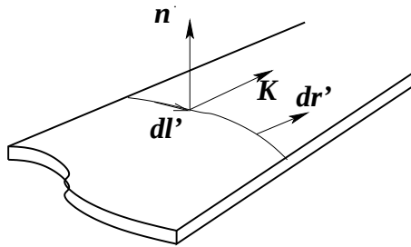
Figura 4.6: También interesan las densidades de corriente superficiales \vec{K} . Integrando \vec{K} a lo largo de una línea transversal se obtiene la corriente total
