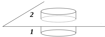
Figura 1.10: Se dibuja una pequeña superficie cilíndrica perpendicular a la superficie de contacto entre los medios "1" y "2".
