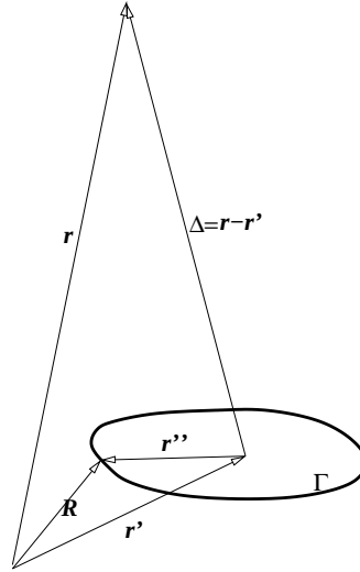
Figura 4.11: Se calcula el potencial lejano \vec{A} asociado a un pequeño circuito \Gamma recorrido por \vec{R} , esto es \|\vec{r}''\| \ll \|\vec{r}\| \approx \|\vec{\Delta}\| .
