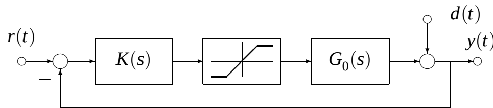
Planta con saturación a la entrada
