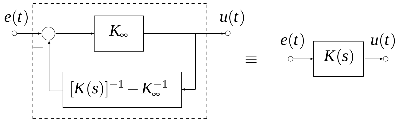
Figura 2: Implementación en realimentación de K(s) bipropia
