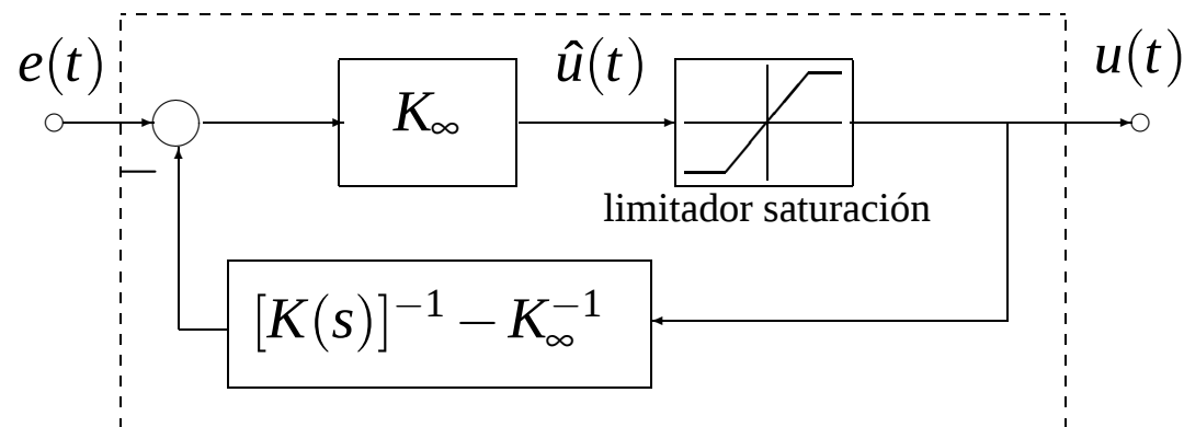
Figura 3: Controlador compensado para saturación
