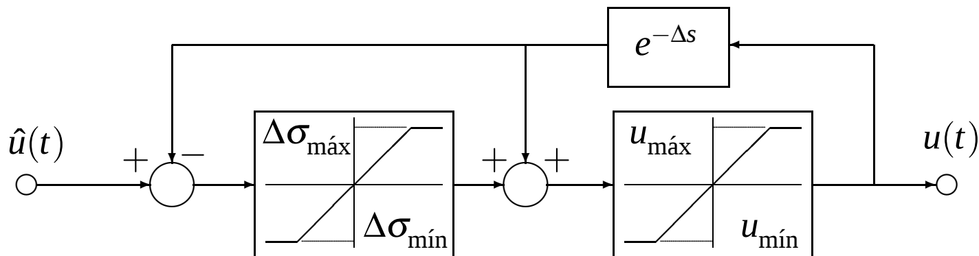
Figura 8: Modelo de limitador combinado saturación- slew rate
