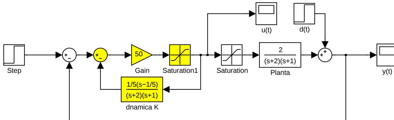
Figura 4: Diagrama Simulink del Ejemplo 2
