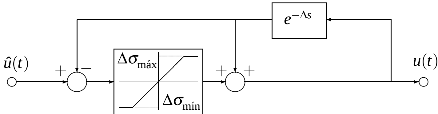
Figura 7: Modelo de limitador slew rate
