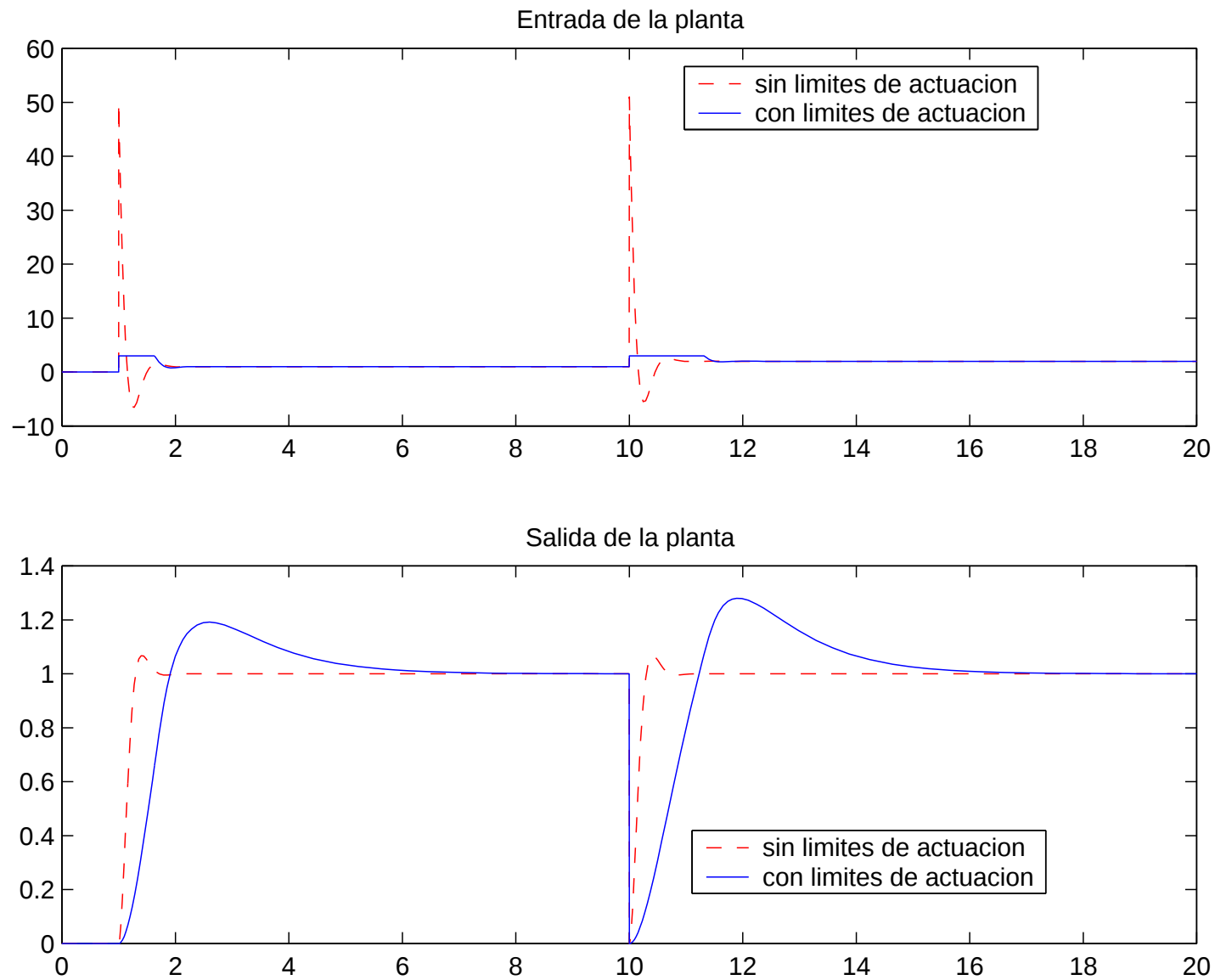
Figura 1: Respuesta con y sin limitaciones de actuación
