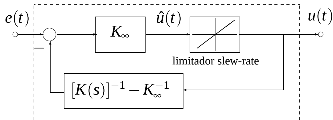
Figura 6: Controlador compensado para slew-rate
