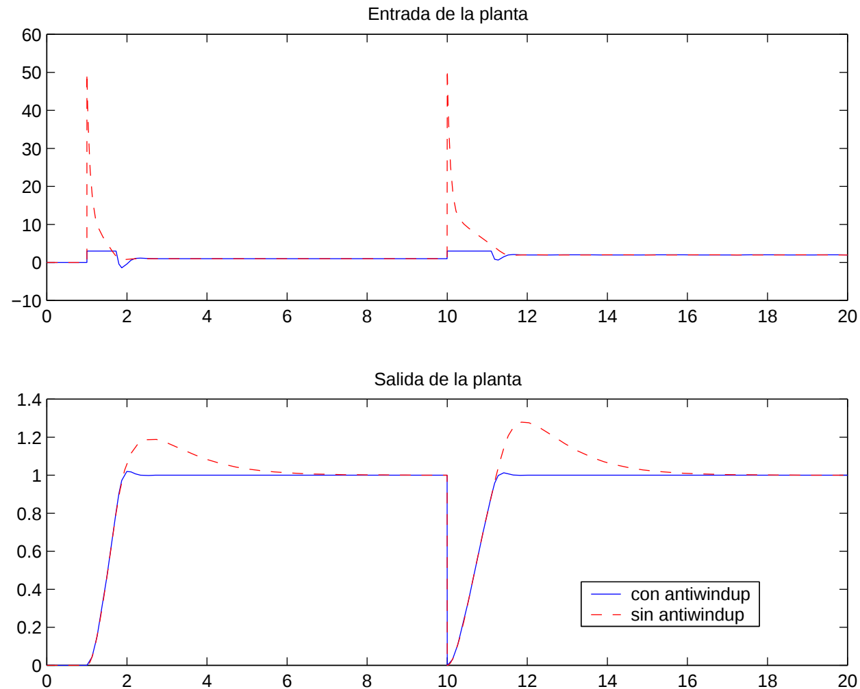
Figura 5: Respuesta del sistema del Ejemplo 2 con y sin AW
