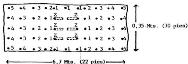
Fig. 15.24 - Diseño normal de retardo con detonadores de medio segundo
