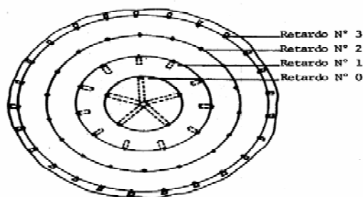
Fig. 15.21 Diseño normal de retardo con detonadores de medio segundo de retardo.
