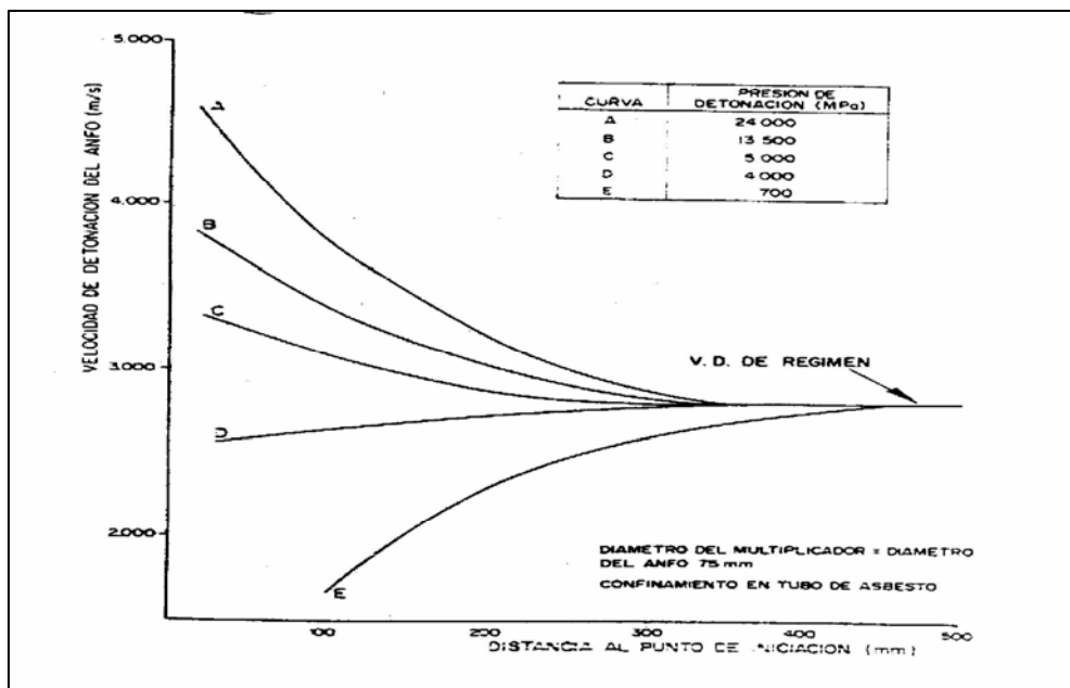
FIGURA 6.1: Efecto de la presión de detonación (PD) del iniciador sobre la VOD del ANFO (Junk,1972) En esta figura observamos una caída de la VOD cuando la PD es inferior a un determinado valor, ocurriendo lo contrario cuando se tiene una PD superior.
