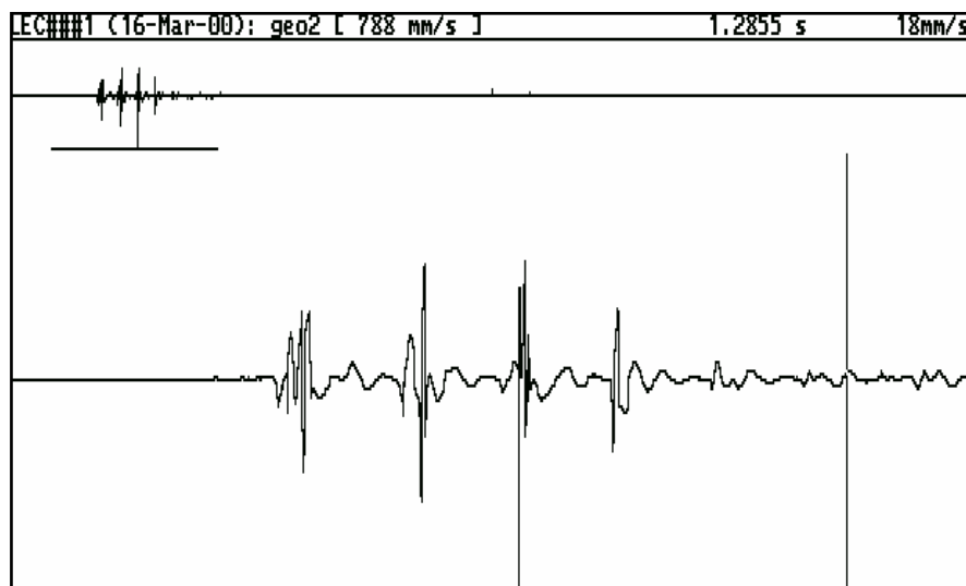
FIGURA 8.5: Registro de vibraciones
