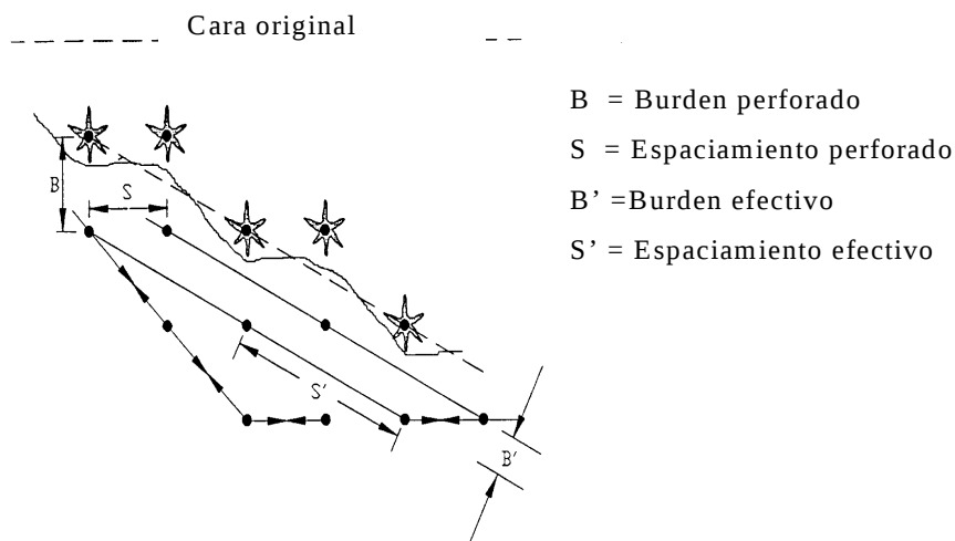
Figura 1.2. Definiciones de burden & espaciamiento nominal y efectivo.
