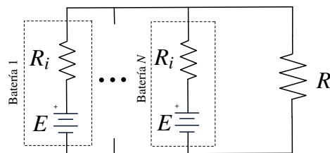
Circuito Paralelo
