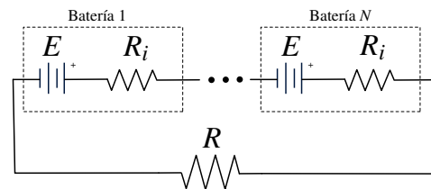
Circuito Serie
