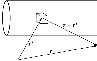
Figura 4.2: Se considera un elemento de volumen en el conductor con corriente. Este pequeño volumen es responsable de una parte d^3\vec{B} del campo total que la corriente provoca.
