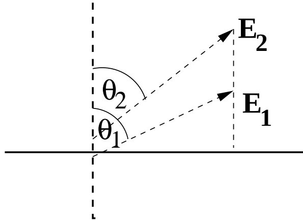
Figura 1.11: La dirección del campo eléctrico a ambos lados de la interfaz entre dos dieléctricos aislantes. (Debe entenderse que ambos campos son evaluados en el mismo punto de la interfaz: cada uno es el límite del valor del campo en el medio respectivo.)
