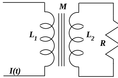
Figura 6.17: Un transformador cuyo secundario está conectado a una resistencia R .
