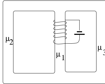
Figura 5.9: Un circuito magnético sencillo.
