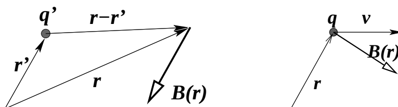
Figura 4.1: A la izquierda una carga q' produce un campo magnético \vec{B}(\vec{r}) en todo punto \vec{r} . A la derecha se tiene la acción de una fuerza magnética sobre una carga en movimiento en presencia de un campo magnético.
