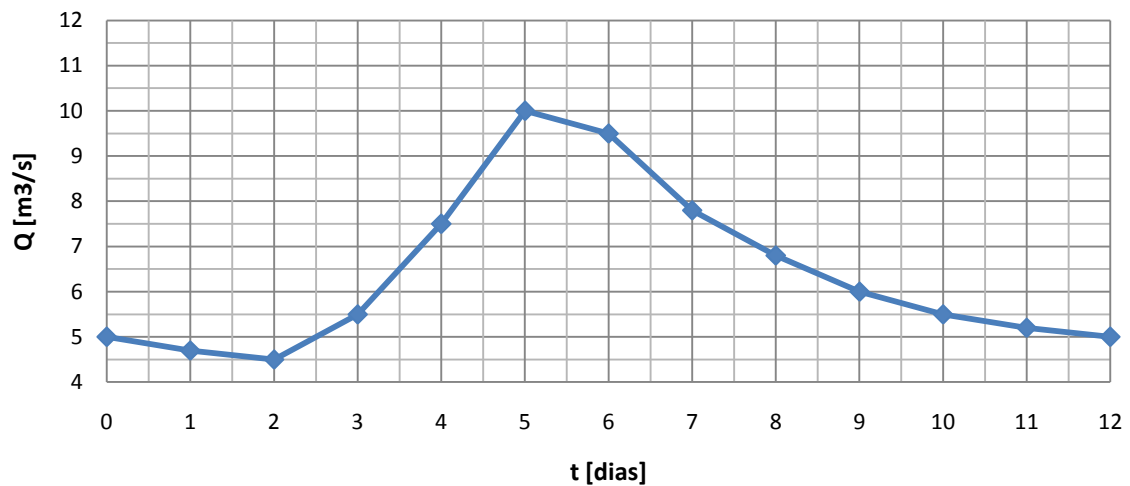
Figura 1: Hidrograma de escorrentía total
