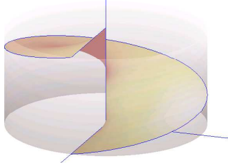
FIGURA 1. Helicoide de radio 1 y altura 1.
