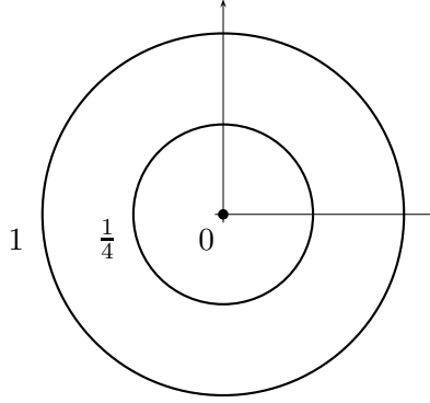
Curvas de nivel para \alpha = 0 , \alpha = \frac{1}{4} y \alpha = 1 .
