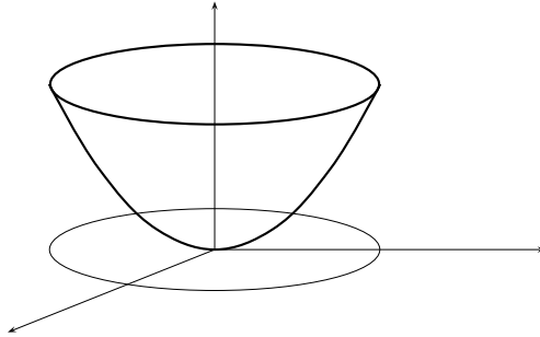
Grafo de f(x, y) = x^2 + y^2 en \Omega .
