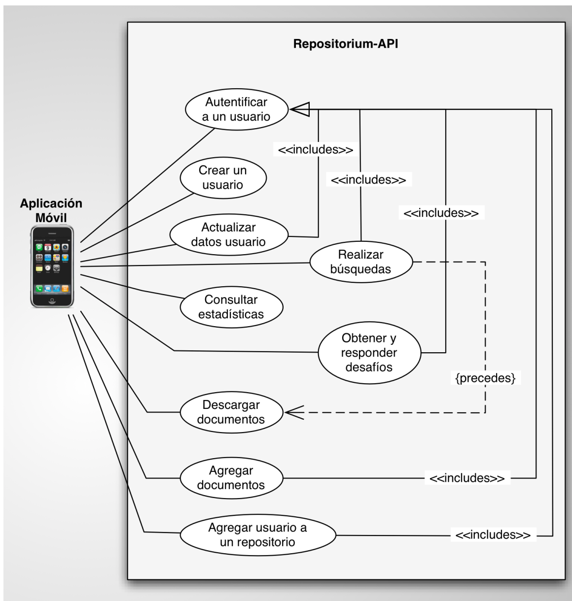
Figura 3: Casos de uso aplicación modelo. Requisitos críticos y deseables
