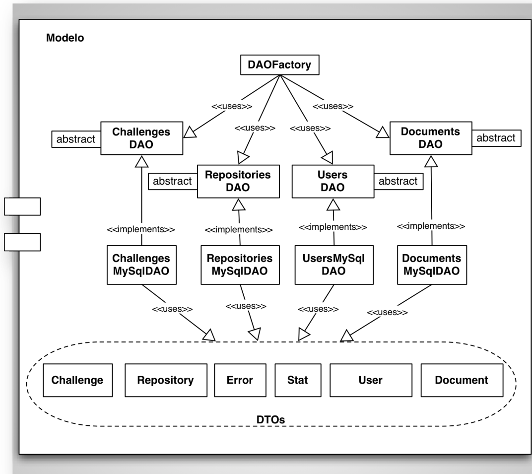
Figura 10: Diagrama de clases, capa Modelo
