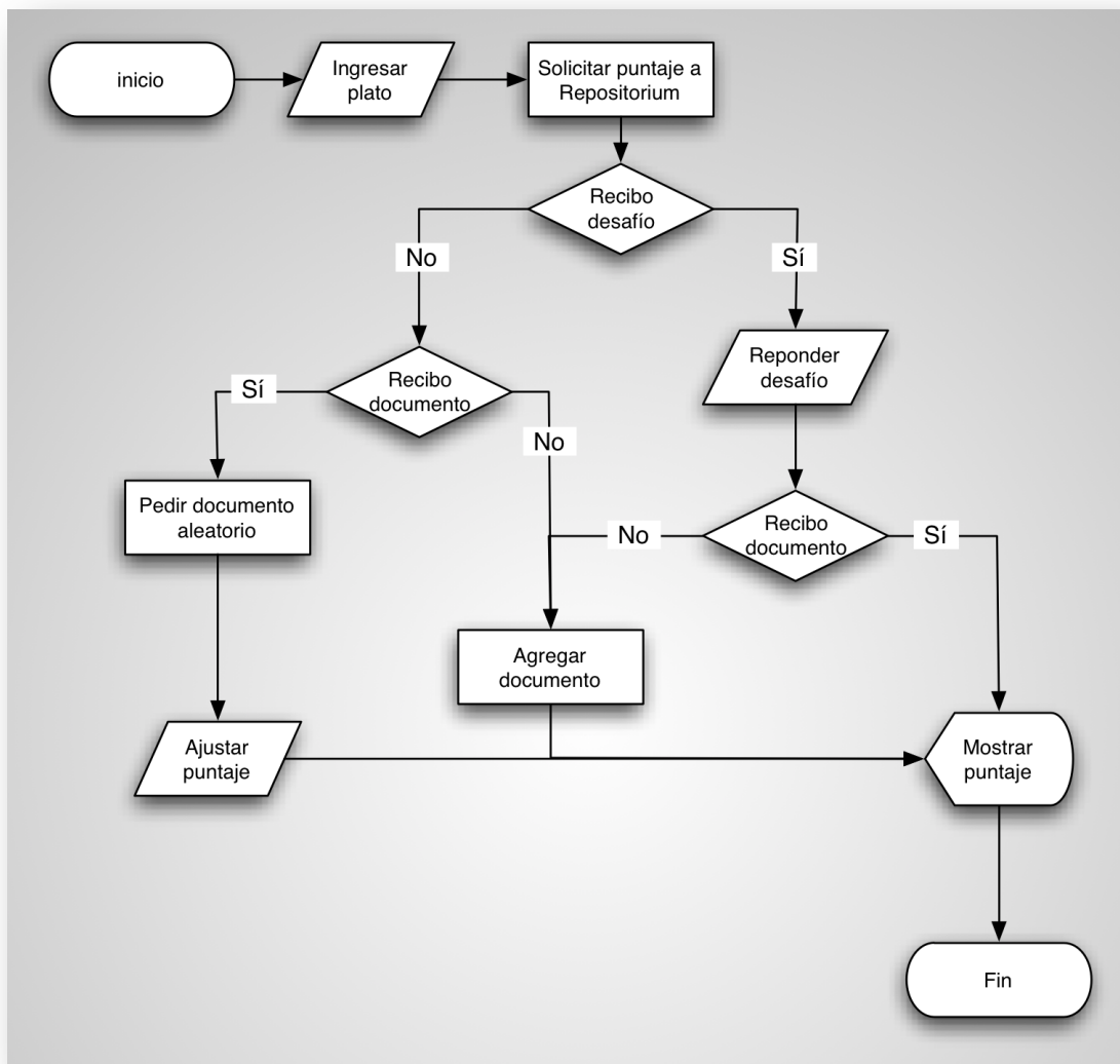
Figura 18: Flujo de navegación con BSDB
