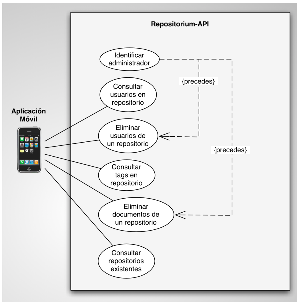
Figura 4: Casos de uso aplicación modelo. Requisitos opcionales
