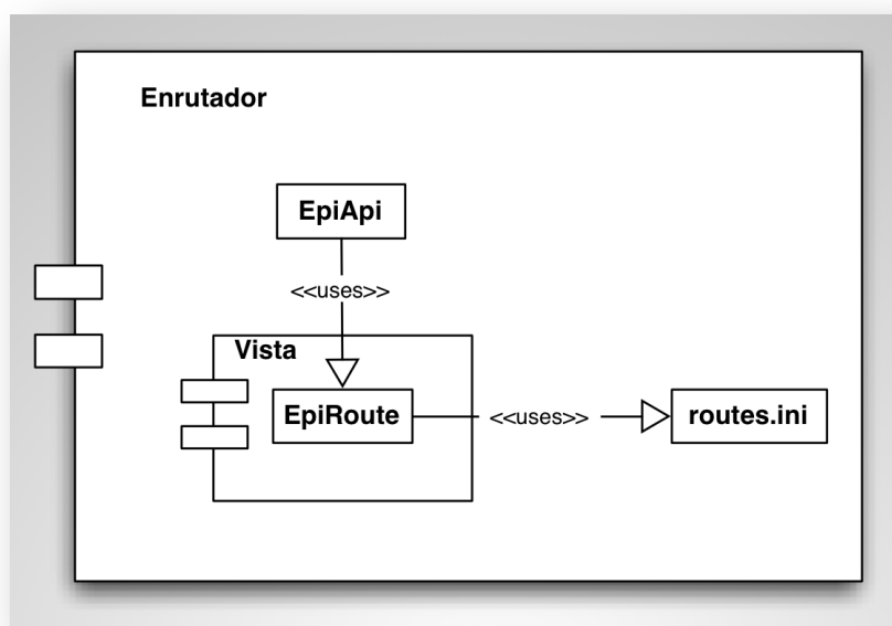
Figura 8: Diagrama de clases, capa Enrutador
