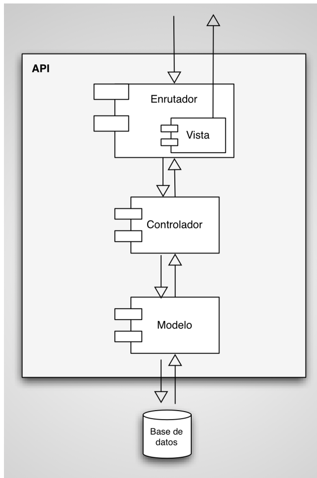
Figura 5: Arquitectura propuesta para la API de Repositorium
