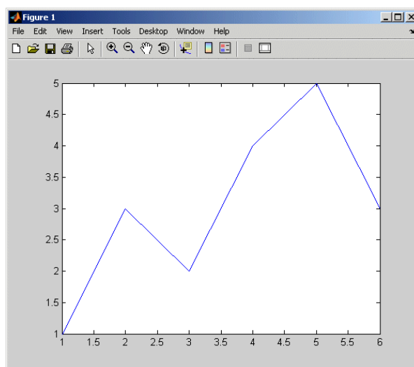
Figura 38. Gráfico del vector x=[1\ 3\ 2\ 4\ 5\ 3] .
