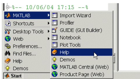
Figura 2. Menú Start/MATLAB.
