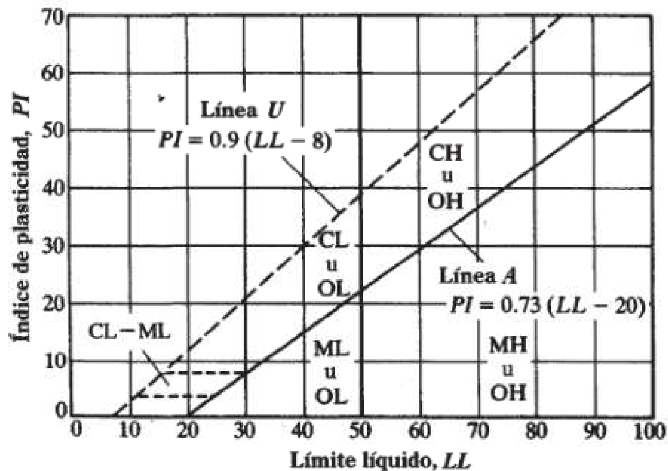
▼ FIGURA 1.7 Carta de plasticidad
