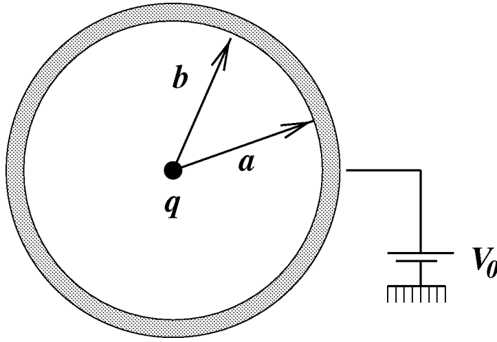
Figura 2.2: Una carga puntual dentro de una esfera conductora hueca
