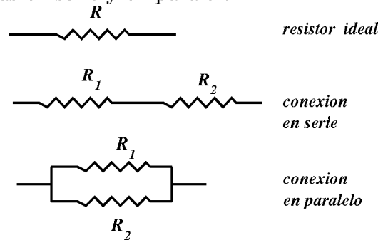
Figura 5.3: Representacion de un resistor ideal, por medio de una línea qeubrada, y de las combinaciones de resistencias en serie y en paralelo.
