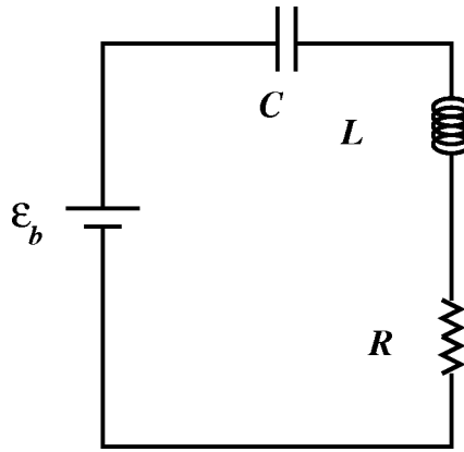
Figura 8.7: Un circuito RLC , con una f.e.m. continua \epsilon_b .
