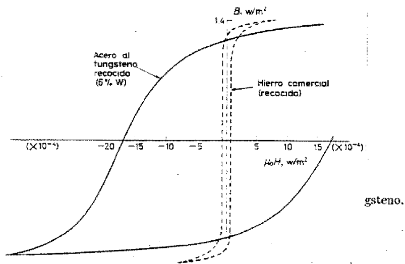
Figura 7.4: Curvas de histéresis para hierro comercial y acero al tungsteno.
