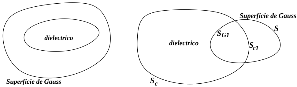
Figura 1.9: Se estudia tanto el caso en que la superficie de Gauss encierra totalmente al dieléctrico aislante como el caso en que solo parte del dieléctrico está dentro de la superficie de Gauss. En la figura de la derecha la superficie de Gauss corta al volumen dieléctrico de modo que carga encerrada por S no es toda la carga del material.
