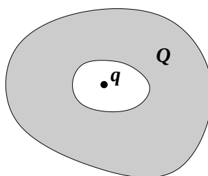
Figura 2.1: Conductor con carga total Q que tiene un hueco que contiene una carga q .
