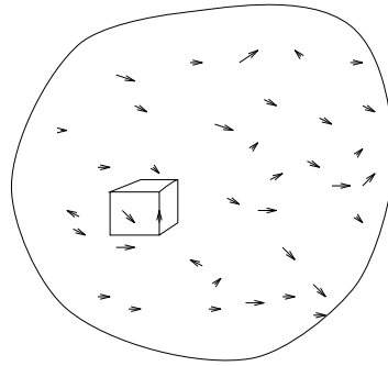
Figura 1.7: Materia compuesta de dipolos moleculares. A cada elemento de volumen diferencial dV se le asocia una polarización \vec{P} tal que el momento dipolar de ese elemento es d\vec{p} = \vec{P} dV
