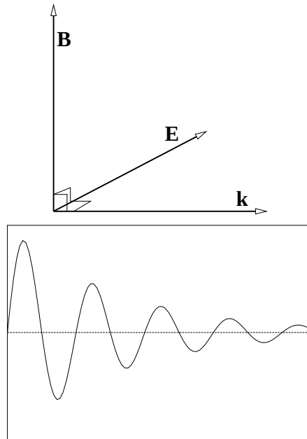
Figura 7.2: En una onda electromagnética la dirección \hat{k} , la dirección del campo eléctrico y la dirección del campo magnético forman una tríada de- recha. La amplitud de la onda disminuye exponencialmente a medida que penetra un medio conductor.
