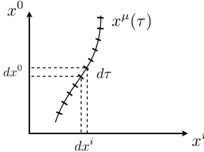
Figure 7: Curva describiendo la trayectoria de una partícula física.
