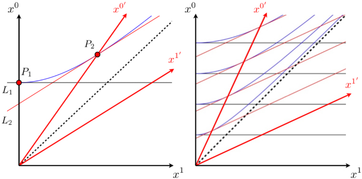
Figure 6: La recta L_1 corresponde al conjunto de eventos simultáneos a P_1 en el sistema inercial del observador O . Así mismo, la recta L_2 corresponde al conjunto de eventos simultáneos a P_2 en el sistema inercial del observador O' . Ambas rectas son tangenciales a la curva invariante \Delta s^2 = -a^2
