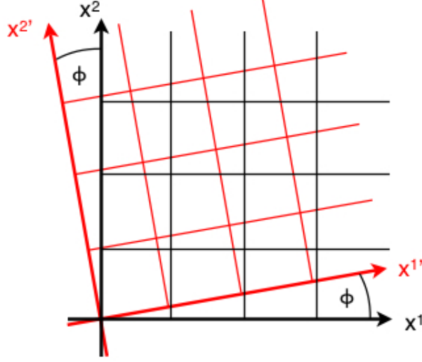
Figure 5: Un caso análogo reconocible es aquel en el cual dibujamos los reticulados de dos sistemas de coordenadas rotados.
