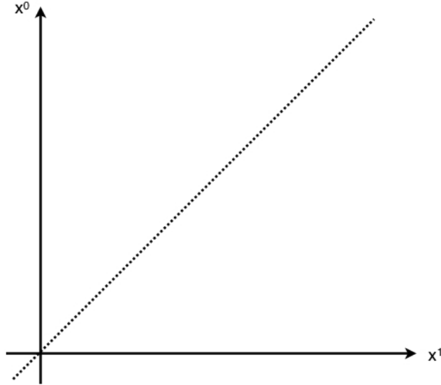
Figure 2: Los ejes t y x del sistema inercial K son perpendiculares el uno con respecto al otro. La figura también muestra la proyección del cono de luz correspondiente a la ecuación t = x .
