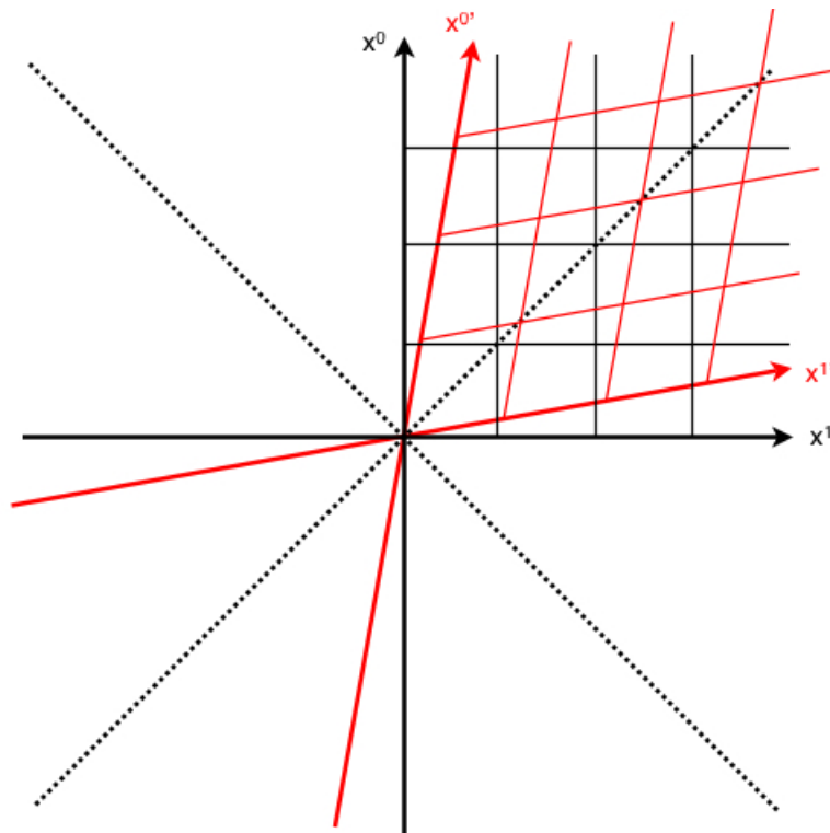
Figure 4: Es posible comparar simultáneamente los cuadriculados de ambos sistemas de coordenadas K y K' . En este caso, hemos optado por un diagrama en el cual los ejes t y x del sistema de coordenadas de K aparezcan perpendiculares.
