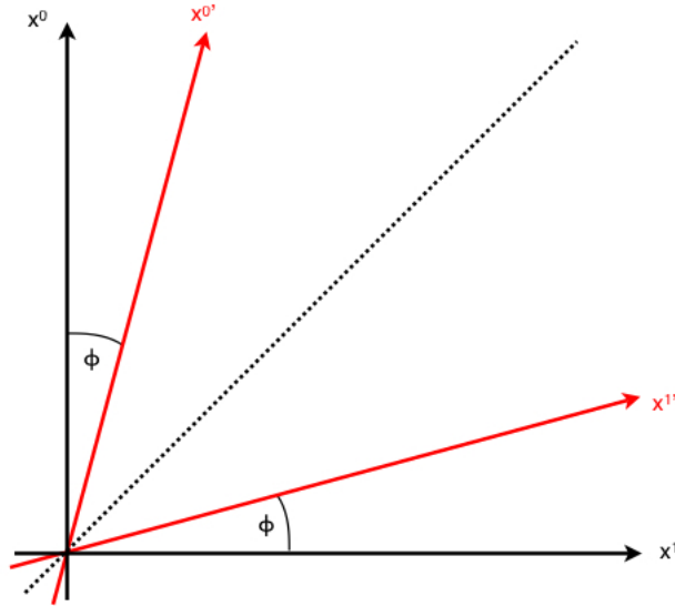
Figure 3: Es posible graficar los ejes t' y x' del sistema K' en el sistema de referencia K . Desde el punto de vista del observador O' , éstos son perpendiculares!
