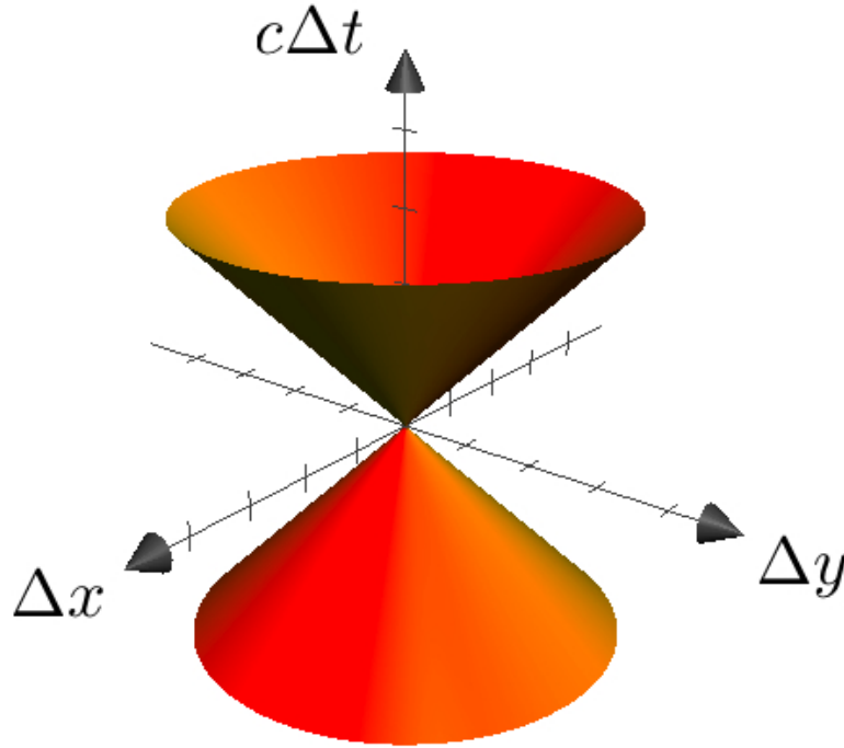
Figure 1: La figura muestra la superficie \Delta s^2 = -c^2(\Delta t)^2 + (\Delta x)^2 + (\Delta y)^2 + (\Delta z)^2 = 0 proyectada sobre el plano (ct, x, y) . Esta superficie es denominada cono de luz.
