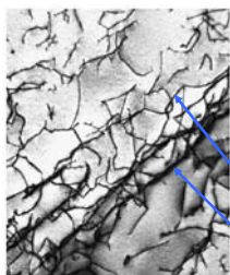
Imagen de dislocaciones por Microscopía Electrónica de Transmisión
