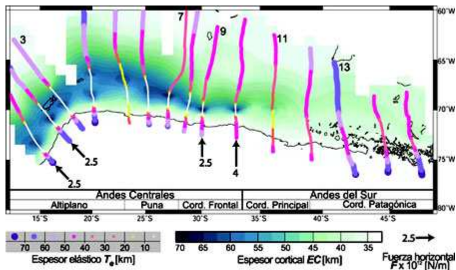
FIG. 4. Presentación de resultados obtenidos por el análisis flexural realizado. Se muestran los valores de espesor elástico a lo largo de cada perfil con círculos que varían de tamaño y color según las variaciones de T_e , la estimación de F a la izquierda de los perfiles donde es distinto de cero ( \times 10^{12} N/m) y un mapa de espesor cortical construido luego de grillar e interpolar los resultados de cada perfil. Perfiles numerados 3, 7, 9, 11 y 13 se presentan en la figura 5 .
