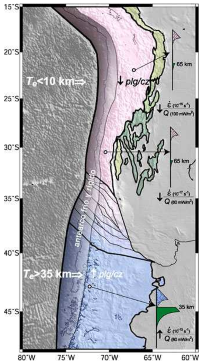
FIG. 8. Interpretación de las variaciones de T_e en el orógeno. Se destaca el contraste composicional entre Andes centrales y del sur, la corteza rica en cuarzo en los Andes centrales limitada al oeste por el antearco rígido y al este por las morfoestructuras del antepaís, la transición composicional a lo largo del segmento Cordillera Principal asociada a estructuras de orientación NW, y las ERDP representativas de los segmentos Altiplano, Cordillera Frontal y Cordillera Patagónica con una estimación de los valores de flujo calórico y tasa de deformación en dichos segmentos (ver texto).
