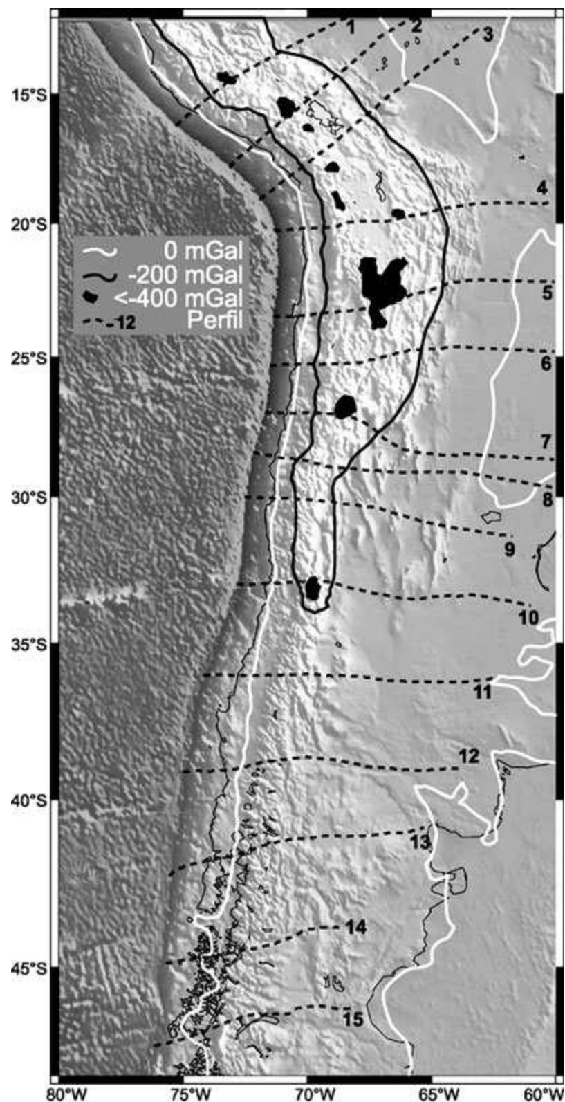
FIG. 2: Isoanomalías de Bouguer 0, -200 y -400 mGal, trazadas sobre la batimetría y topografía blanco y negro. Líneas segmentadas numeradas de 1 al 15 representan los perfiles utilizados en la modelación flexural realizada.
