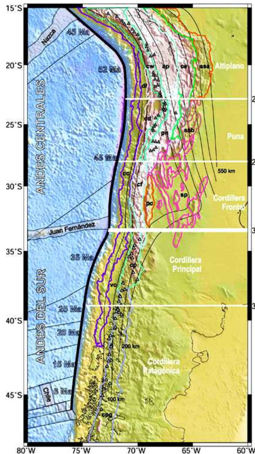
FIG. 1. Características geotectónicas del sistema de convergencia andino entre 15 y 47°S, sobre batimetría y topografía color del área. Unidades morfoestructurales delimitadas por líneas de colores y rotuladas como sigue: cc - Cordillera de la Costa; di - Depresión Intermedia; cw - Cordillera Occidental; ap - Cordillera Oriental; ce - Sierras Subandinas; cd - Cordillera Domeyko; pn - Puna; ssb - Sistema de Santa Bárbara; cf - Cordillera Frontal; sp - Sierras Pampeanas; vc - Valle Central; cp - Cordillera Principal; cpg - Cordillera Patagónica. Triángulos grises y blancos representan los volcanes de la Zona Volcánica Central (ZVC) y Sur (ZVS), respectivamente. Líneas delgadas representan las curvas de profundidad de la placa subductada ( Cahill e Isacks, 1992 ; Craeger et al., 1995 ). Línea gruesa es la fosa Perú-Chile. Números a la izquierda de la fosa denotan la edad de la placa de Nazca. Se destacan las dorsales y zonas de fractura principales de dicha placa. En color blanco se destacan los límites y nombres propuestos (ver texto) de los segmentos de primer orden (mayúsculas izquierda) y segundo orden (minúsculas derecha) en el área de estudio.
