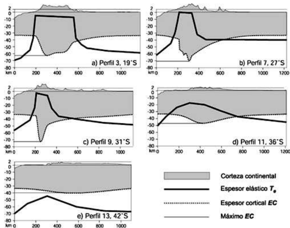
FIG. 5. Perfiles representativos de cada segmento estudiado. Ellos muestran la topografía, el espesor elástico estimado (línea continua gruesa), el espesor cortical calculado (línea punteada) y el máximo espesor cortical (línea continua delgada). Eje horizontal es la distancia en km desde la fosa. En el eje vertical, la topografía sobre el nivel del mar tiene una exageración 2:1 con respecto a la profundidad bajo el nivel del mar.
