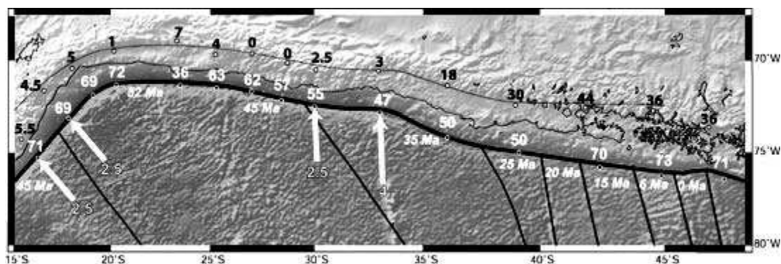
FIG. 7. Resultados y antecedentes utilizados en la interpretación de los mismos en el sector antearco. Se destacan los valores extremos de T_e para cada perfil (máximo en la fosa en blanco, mínimo en el eje del orógeno en negro), los valores de F distintos de cero ( \times 10^{12} N/m), la edad de la placa de Nazca en la fosa y la curva de 100 km de profundidad de la losa subductada bajo el antearco.
