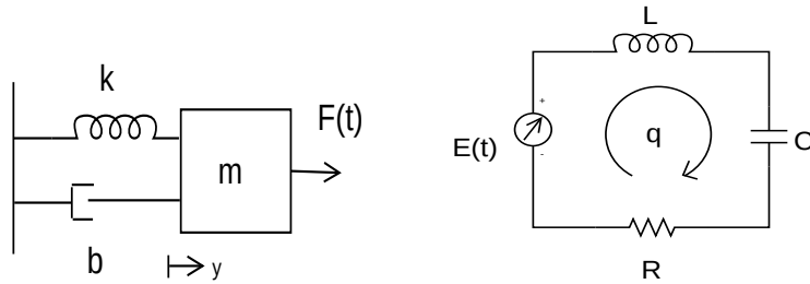
FIGURA 1. Analogía electromecánica.
