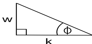
FIGURA 4. Relación entre \phi , k y \omega .
