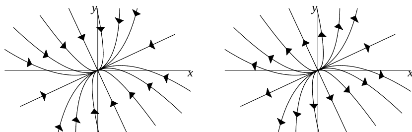
FIGURA 16. Diagramas de fase de (48) para \lambda_2/\lambda_1 > 1 .
