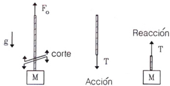
Figura III.1: La Tercera Ley de Newton en acción. F_0 representa la fuerza que se aplica sobre el bloque a través de la cuerda. El tipo que sujeta la cuerda soporta una fuerza -F_0 . Al cortar esta cuerda, en forma imaginaria, debemos reemplazar en cada extremo cortado la tensión T de acuerdo a esta ley.
