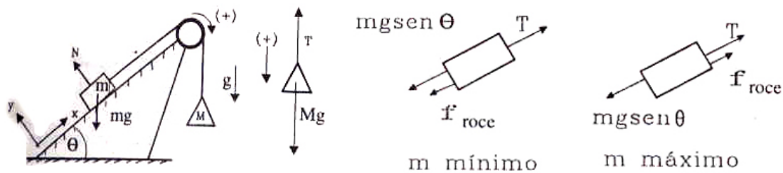
Figura III.31: La fuerza de roce se opone al inicio del movimiento hasta que alcanza un valor límite igual a \mu N . En el primer caso apunta hacia el vértice inferior del plano ( m mínimo). En el segundo caso invierte su sentido.
