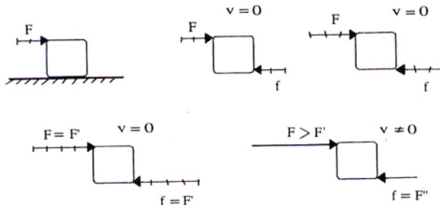
Figura III.27: A medida que la fuerza horizontal F aumenta en magnitud, también lo hace la fuerza de roce f , hasta que llega a su cota máxima F' . Cuando F se hace mayor que este valor F' , el bloque comienza a moverse y el roce estático se transforma en roce cinético.
