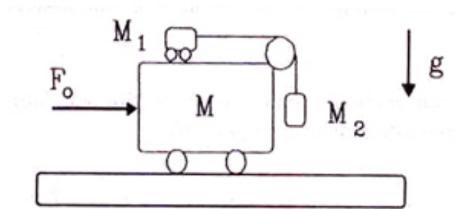
Figura III.17: En este problema debemos encontrar el valor de la fuerza que le comunica al sistema una aceleración igual a la que experimenta la masa M_1 que va montada sobre el carro. La aceleración de ésta última se debe al peso de M_2 .
