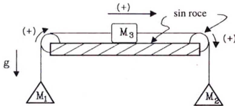
Figura III.11: Este problema incorpora la masa de la cuerda –a través de M_3 – a la dinámica de las masas del ejemplo anterior. Hemos reemplazado la cuerda por una masa puntual para evitar el análisis de la variación de masa debido al movimiento de la cuerda en los costados.
