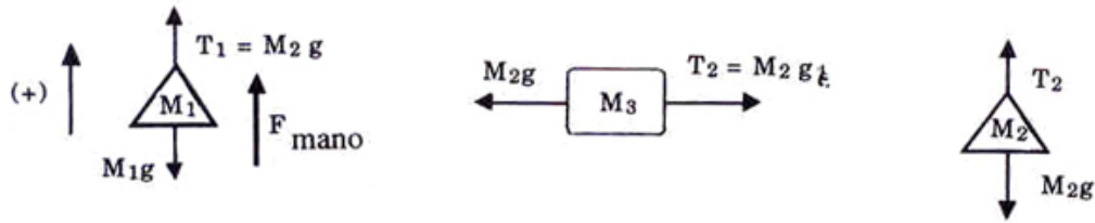
Figura III.15: Diagrama de fuerzas correspondientes al caso c) para cada una de las masas.
