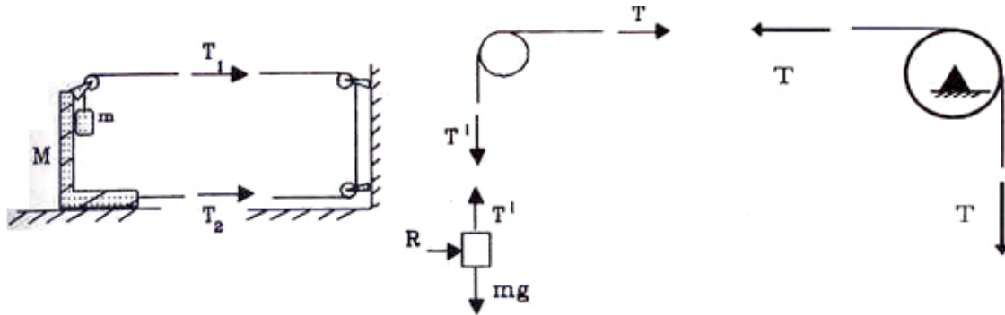
Figura III.20: Aquí se incluye el sistema original y los diagramas de cuerpo libre de la masa M y m . La Figura muestra que si la masa M avanza, digamos 1 cm hacia la derecha, la distancia que recorre el hilo entre la masa M y la pared se acorta en 2 cm y, en consecuencia, la masa m baja 2 cm.
