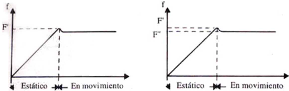
Figura III.28: Se incluye un gráfico del valor con el cual la fuerza de roce responde a una fuerza externa. El movimiento comienza cuando se alcanza el valor F' . Posteriormente la fuerza de roce cambia y se estabiliza en el valor F'' , correspondiente al roce cinético.
