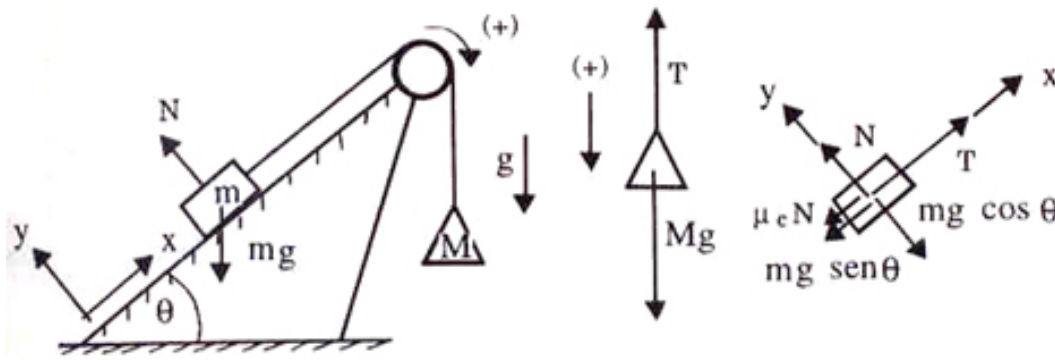
Figura III.30: A cada una de las masas le asociamos una fuerza que corresponde a su peso. Sobre m actúa la reacción del piso que se descompone en una fuerza normal al piso y otra tangente que identifica a la fuerza de roce.
