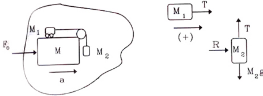
Figura III.18: Se incluye a la izquierda el diagrama de cuerpo libre de el sistema considerado como un todo . A la derecha aparecen los diagramas de cuerpo libre de las masas M_1 y M_2 .
