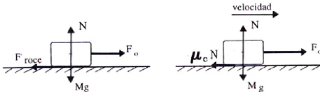
Figura III.29: Se muestra el diagrama de cuerpo libre y la definición de la fuerza de roce con el coeficiente de roce estático (antes de que se produzca el movimiento) y el roce cinético , en el caso de un bloque deslizando sobre una superficie rugosa.
