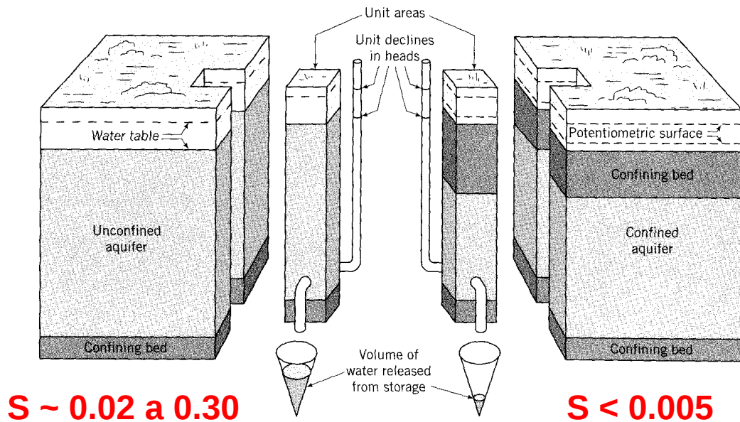
Figura 4.2 Coeficiente de Almacenamiento para Formaciones Acuíferas Libres y Confinadas
