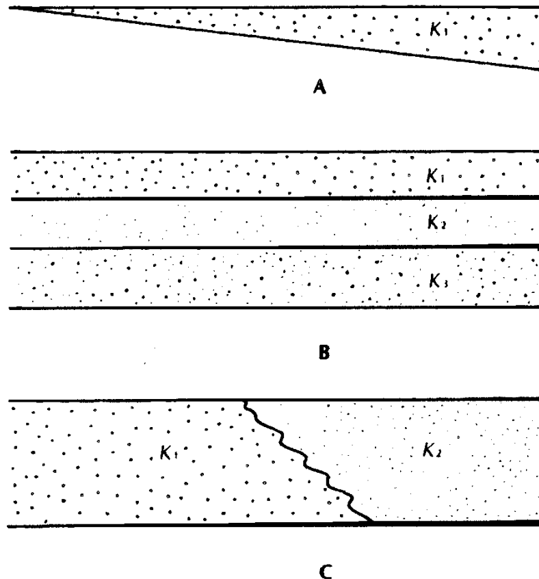
Figura 3.1 Ejemplo de Formaciones Acuíferas Heterogéneas
