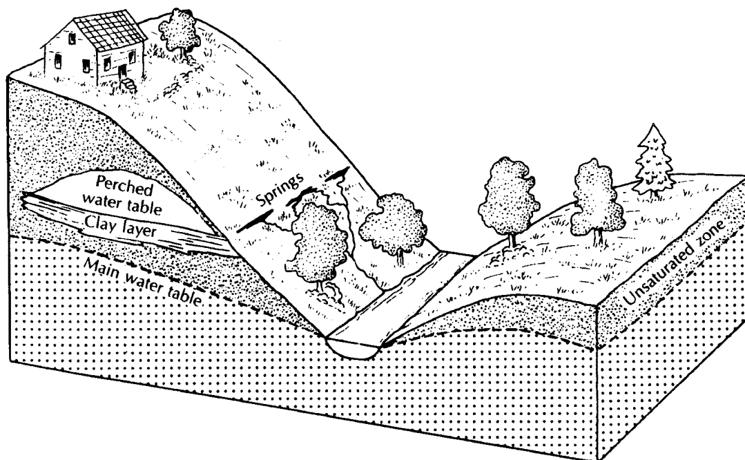
Figura 2.4 Acuífero Colgado
