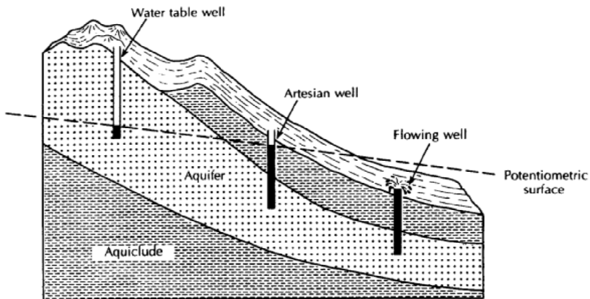
Figura 2.3 Nivel Piezométrico y Tipos de Pozos
