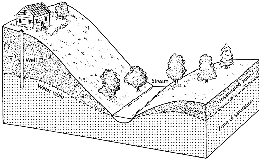
Figura 2.1 Acuífero No Confinado o Libre
