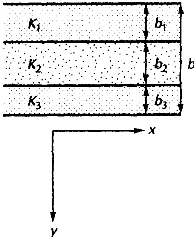
Figura 3.4 Ejemplo de Sistema Estratificado
