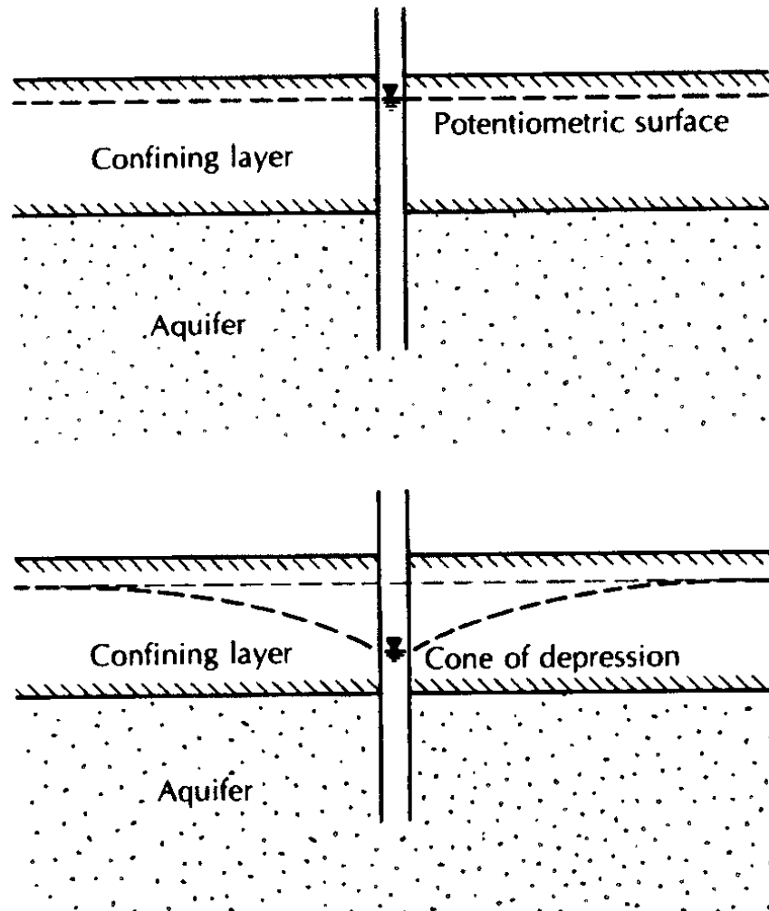
Figura 4.1 Liberación de Agua en un Acuífero Confinado
