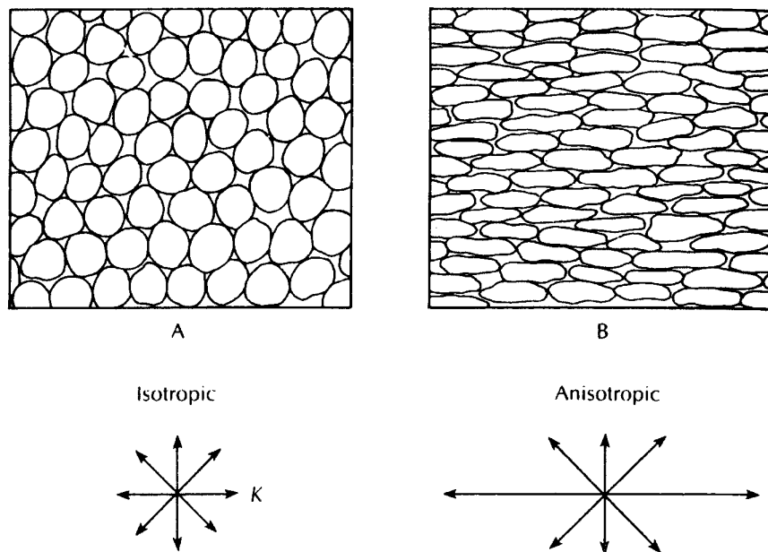
Figura 3.2 Formaciones Acuíferas Isotrópicas y Anisotrópicas
