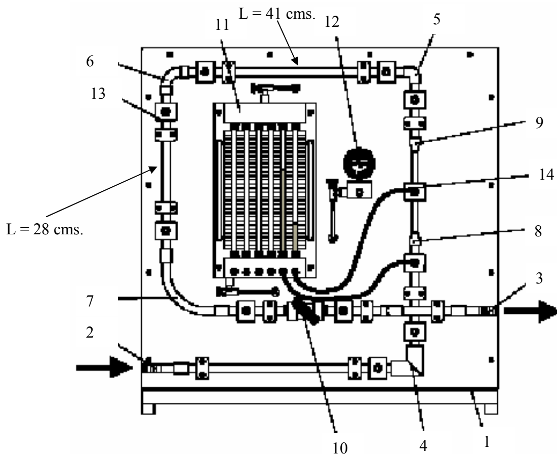
Figura 1.1. Instalación Experimental.
