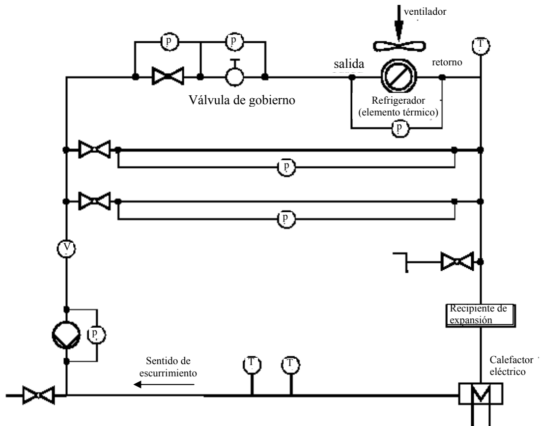
Figura 3A.2. Esquema del Circuito de Agua.
