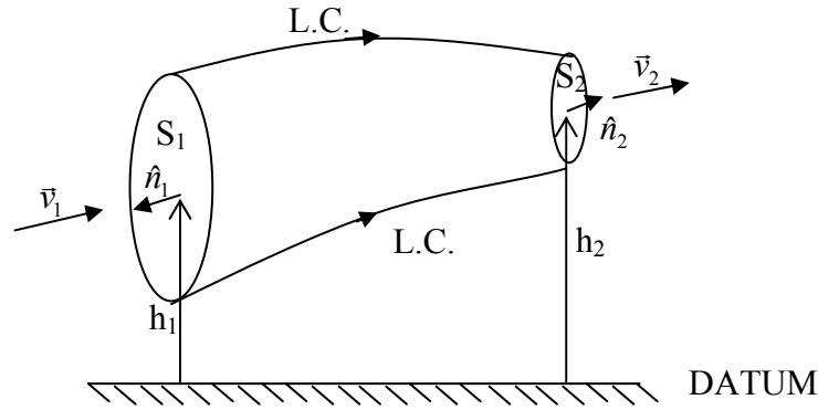
Figura 3A.1. Volumen de Control
