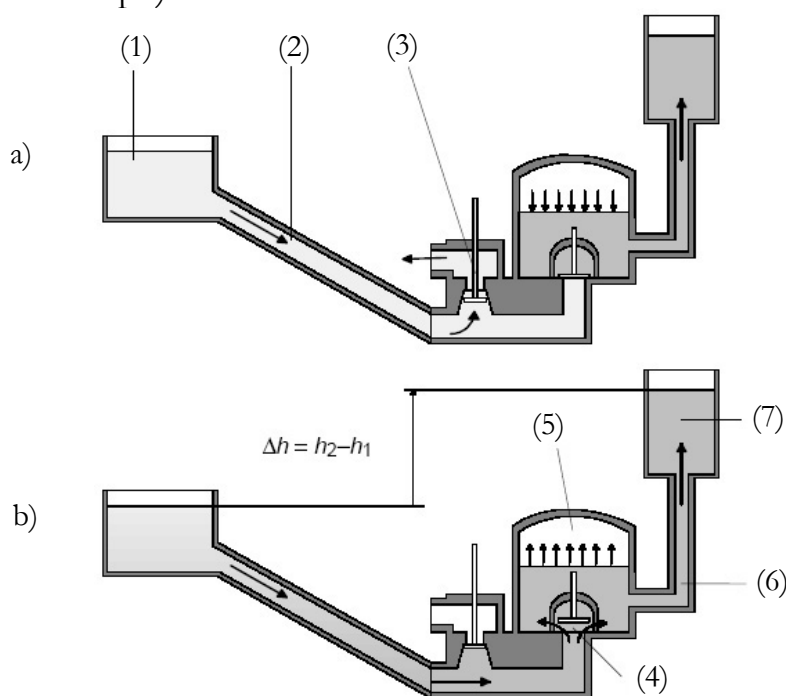
Figura 3B.2. Esquema de bomba de ariete hidráulico.
