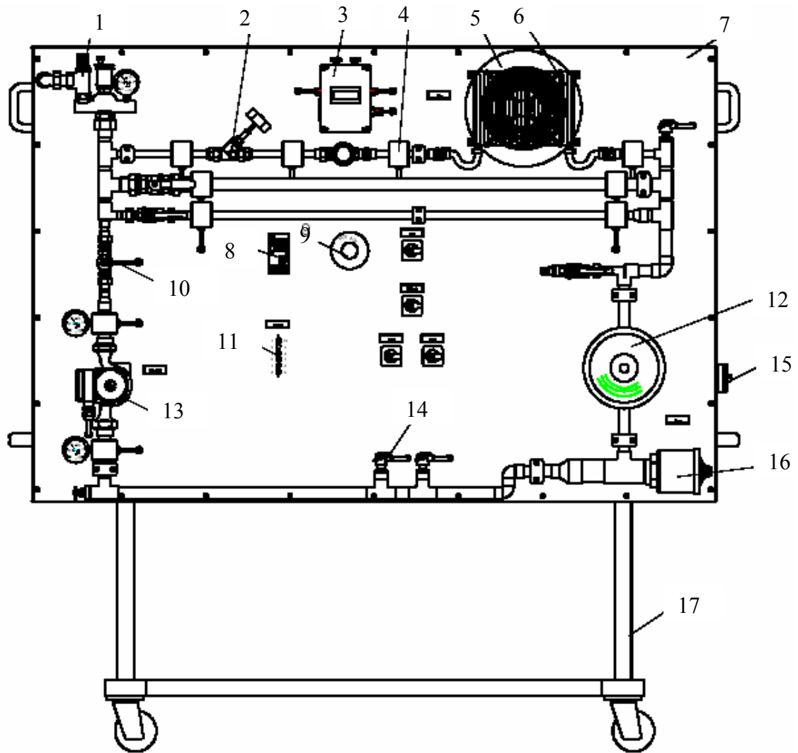
Figura 3A.3. Estructura del Equipo.
