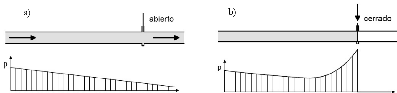
Figura 3B.1. Esquema de variación de presiones por el cierre brusco de una válvula.
