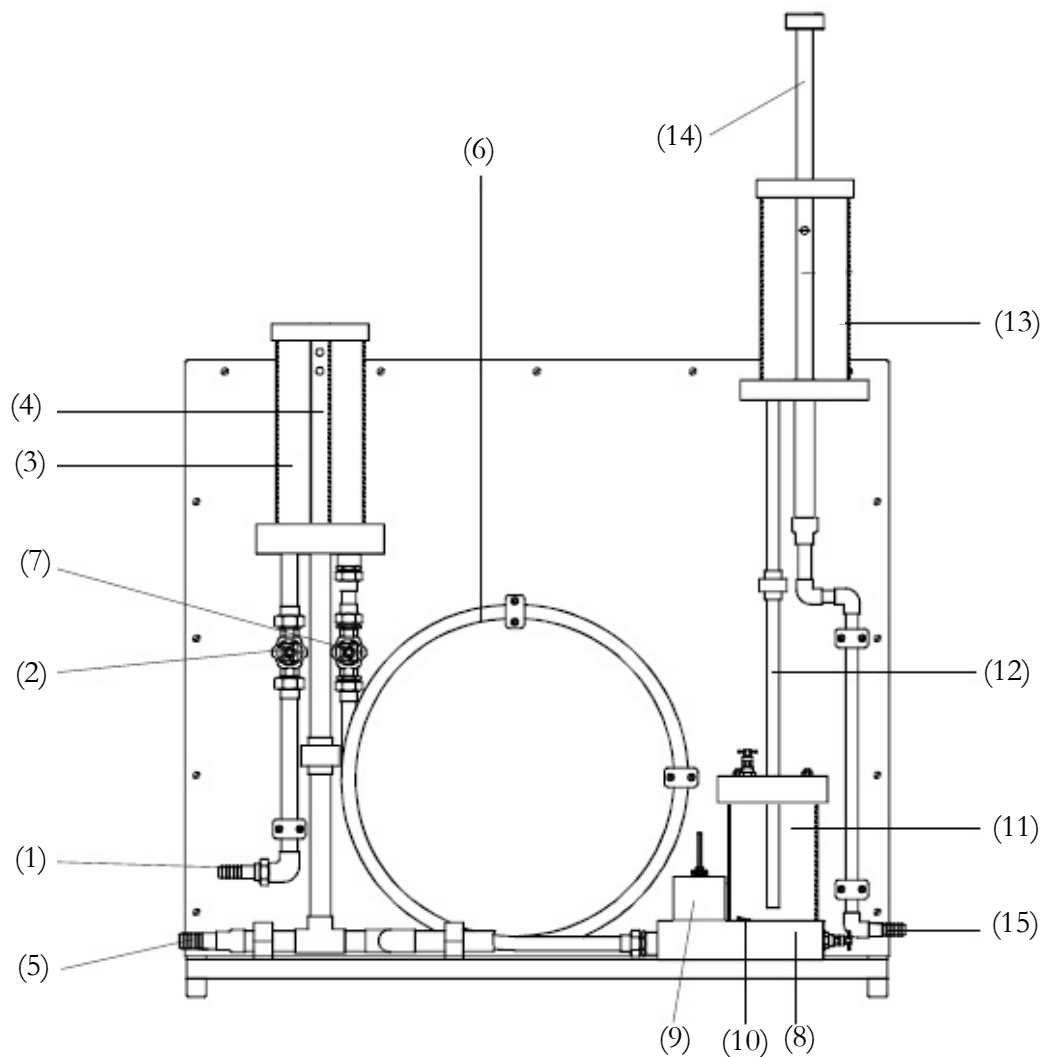
Figura 3B.3. Instalación Experimental
