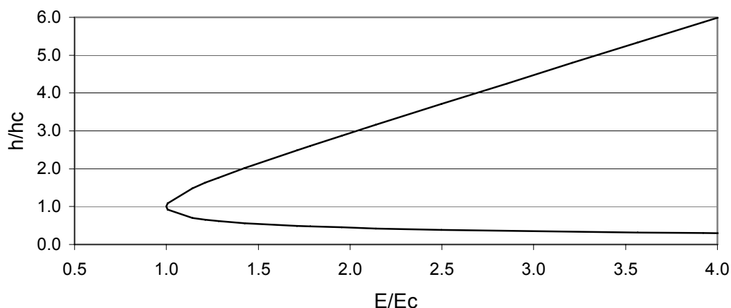
Figura 4.2. Curva de Energía Específica en Canales Rectangulares.
