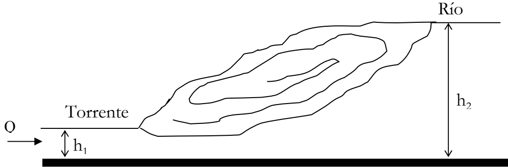
Figura 4.4. Resalto Hidráulico.
