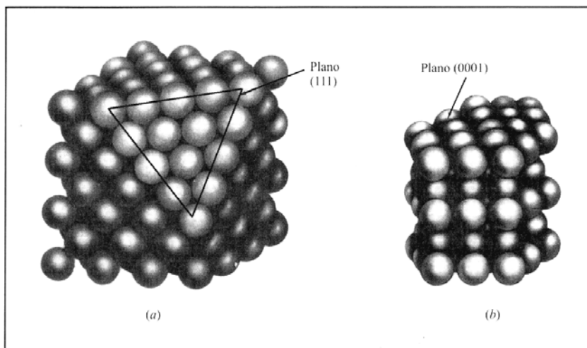
Figura 3.19. Comparación de (a) la estructura cristalina FCC mostrando planos (111) de empaquetamiento compacto y (b) de la estructura cristalina HCP mostrando planos de empaquetamiento compacto (0001). (Según W. G. Moffat, G. W. Pearsall y J. Wulff, «The Structure and Properties of Materials», vol. 1: «Estructura», Wiley, 1964, pág. 51.)
