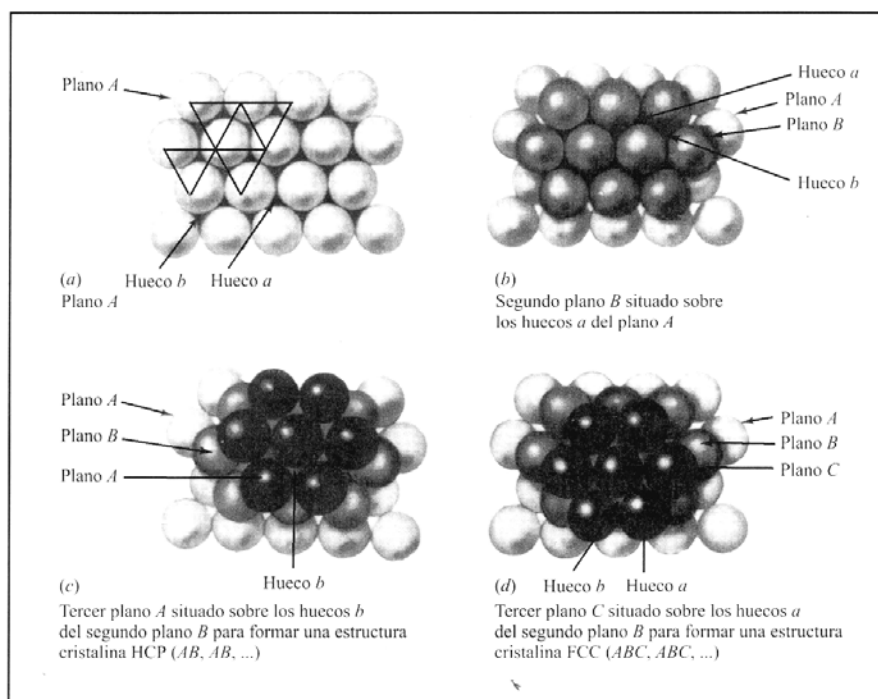
Figura 3.20. Formación de las estructuras cristalinas HCP y FCC por apilamiento de planos de empaquetamiento compacto de átomos. (a) Plano A conteniendo huecos de tipo a y b entre átomos. (b) Plano B colocado sobre los huecos a del plano A. (c) Tercer plano: otro plano A colocado sobre los huecos b del segundo plano B formando la estructura cristalina HCP (ABABAB...). (d) Tercer plano: un plano C es colocado sobre los huecos a del plano B formando una estructura cristalina FCC de apilamiento ABCABC...
