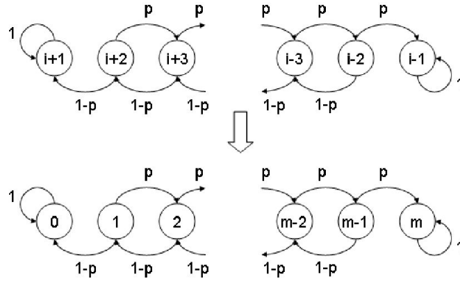
Figura 2: Analogía cálculo de “visita primero”
