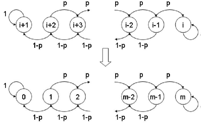
Figura 3: Analogía “primero i-1 ”
