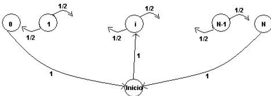
Figura 1: grafo asociado a la P2
