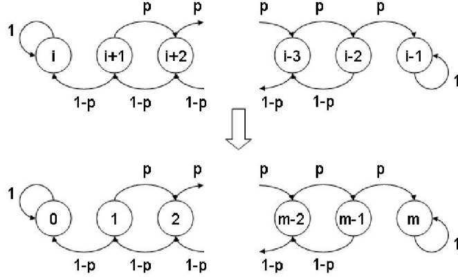
Figura 4: Analogía “primero i + 1 ”
