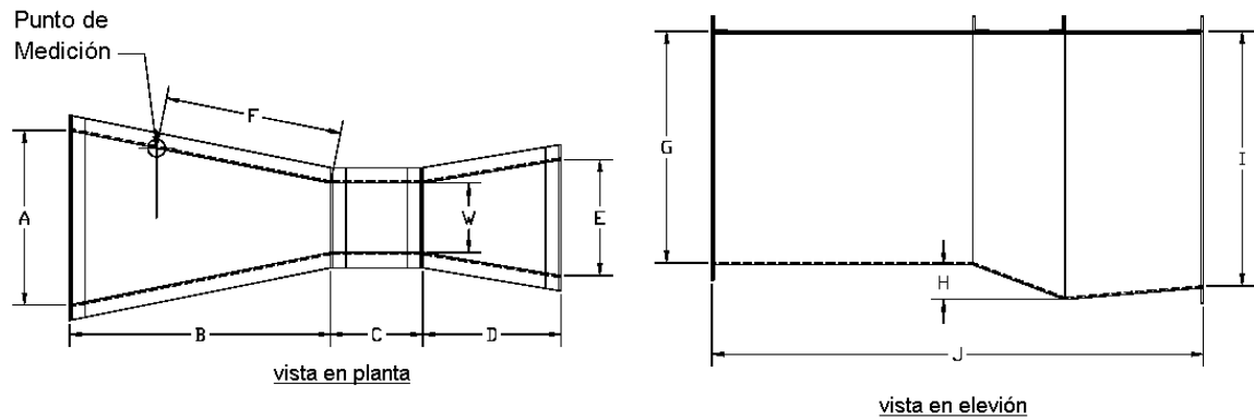
Figura 4.1: Características y medidas de Canaletas Parshall
