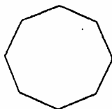
(9) Ditetragonal prism
