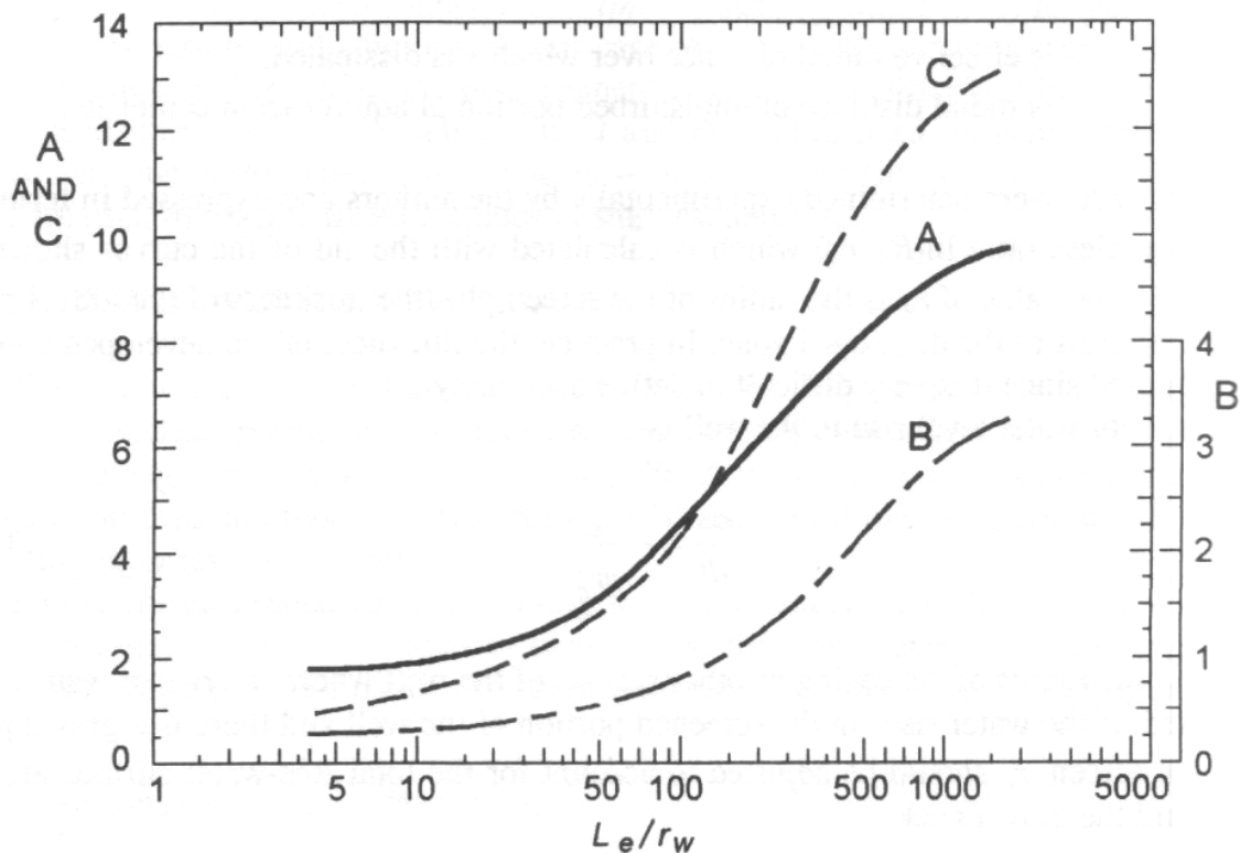
Figura 2.2 Parámetros Adimensionales A, B y C (Bouwer and Rice)
