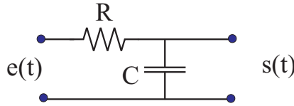
Figura 2.12: Integrador analógico
