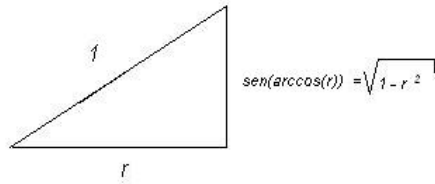
Figura 2: Simplificación de \sin(\arccos(r))
