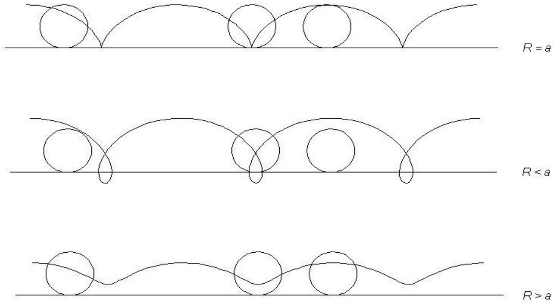
Figura 1: Cicloide
