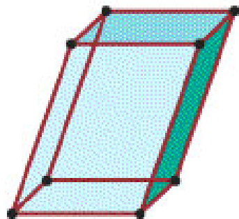
Monoclinic
