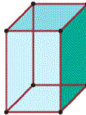
Orthorhombic
