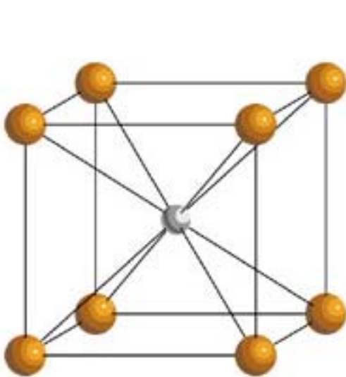
CsCl
