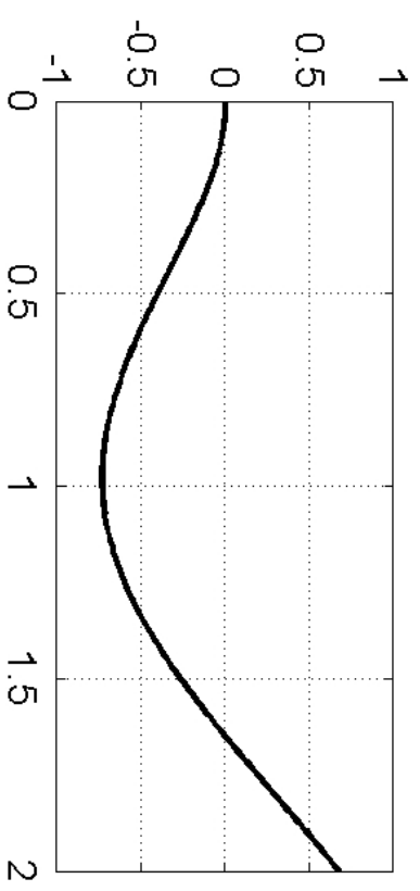
\phi_2(x)
