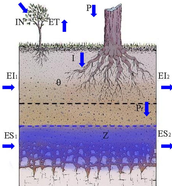
Fig. 1.2: Esquema del subsistema suelo - agua - planta
