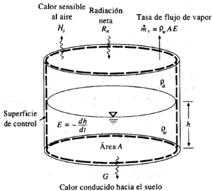
Fig. 1.3: Volumen de control en un tanque de evaporación definido para el cálculo de la evaporación (Fuente: Chow et al. 1994).
