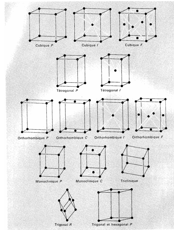
Figure 14 Les quatorze réseaux de Bravais. Les mailles figurées sont les mailles conventionnelles qui ne sont pas toujours élémentaires.
