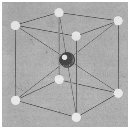
Fig. 15 Celda cristalina del CsCl
