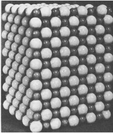
Fig. 12 Modelo del cristal iónico NaCl
