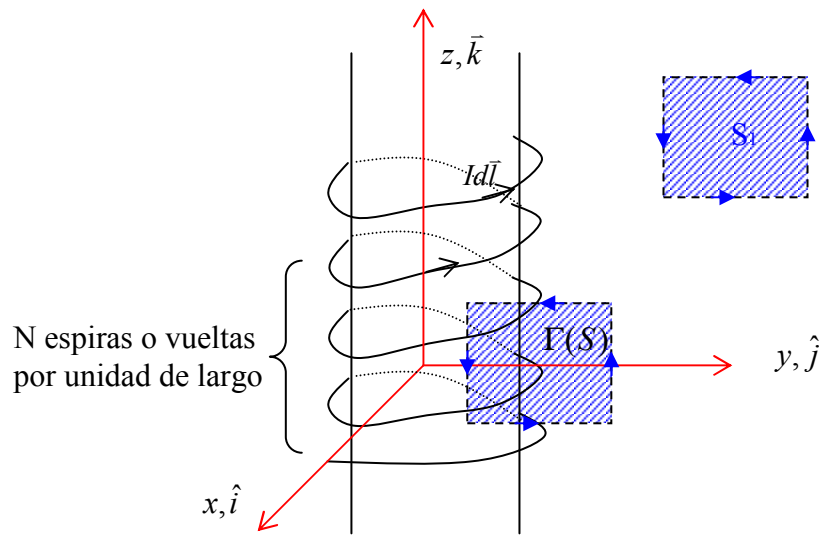
Figura 133. Campo bobina.
