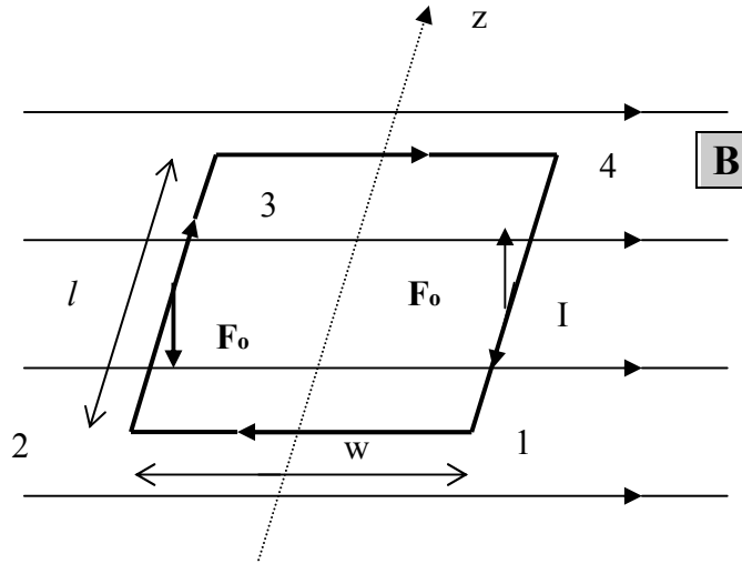
Figura 131. Torque magnético.
