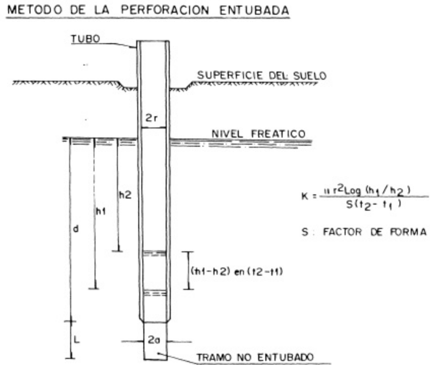
Figura 2.2 Factor de Forma S en Prueba en Perforación Entubada
