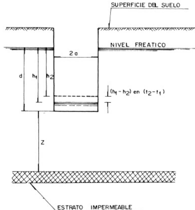
Figura 3.1 Prueba en Perforación No Entubada
