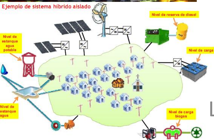
Ejemplo de sistema híbrido aislado
