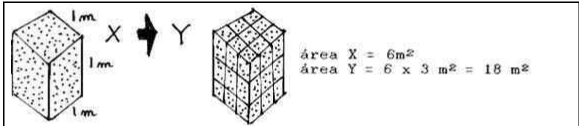
Figura 36. Bloque fracturado merced a un sistema de diaclasas. Las fracturas son ortogonales y de igual espaciado. Se observa cómo el fracturamiento ofrece más área de exposición pues si el bloque X tiene 6 m 2 , la formación de pequeños bloques con aristas 3 veces más pequeñas, triplicará el área de exposición. Adaptado de Leet y Judson, Geología física.
