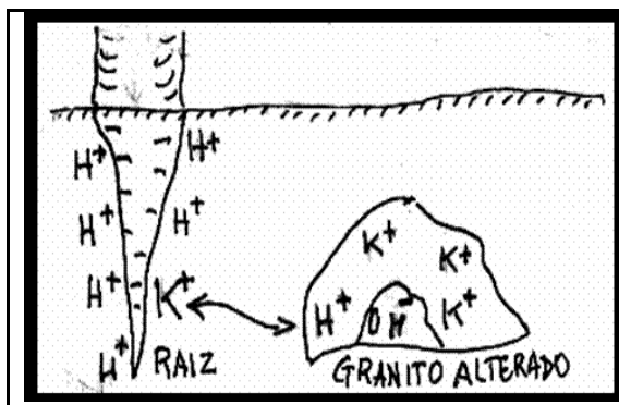
Figura 37. Raíz de una planta formando arcillas. Por las cargas eléctricas (-) de la raíz hay adherencia de iones de hidrógeno (H + ); la ortoclasa tendrá disponible iones de potasio (K + ). Adaptado de Leet y Judson, Geología física.
