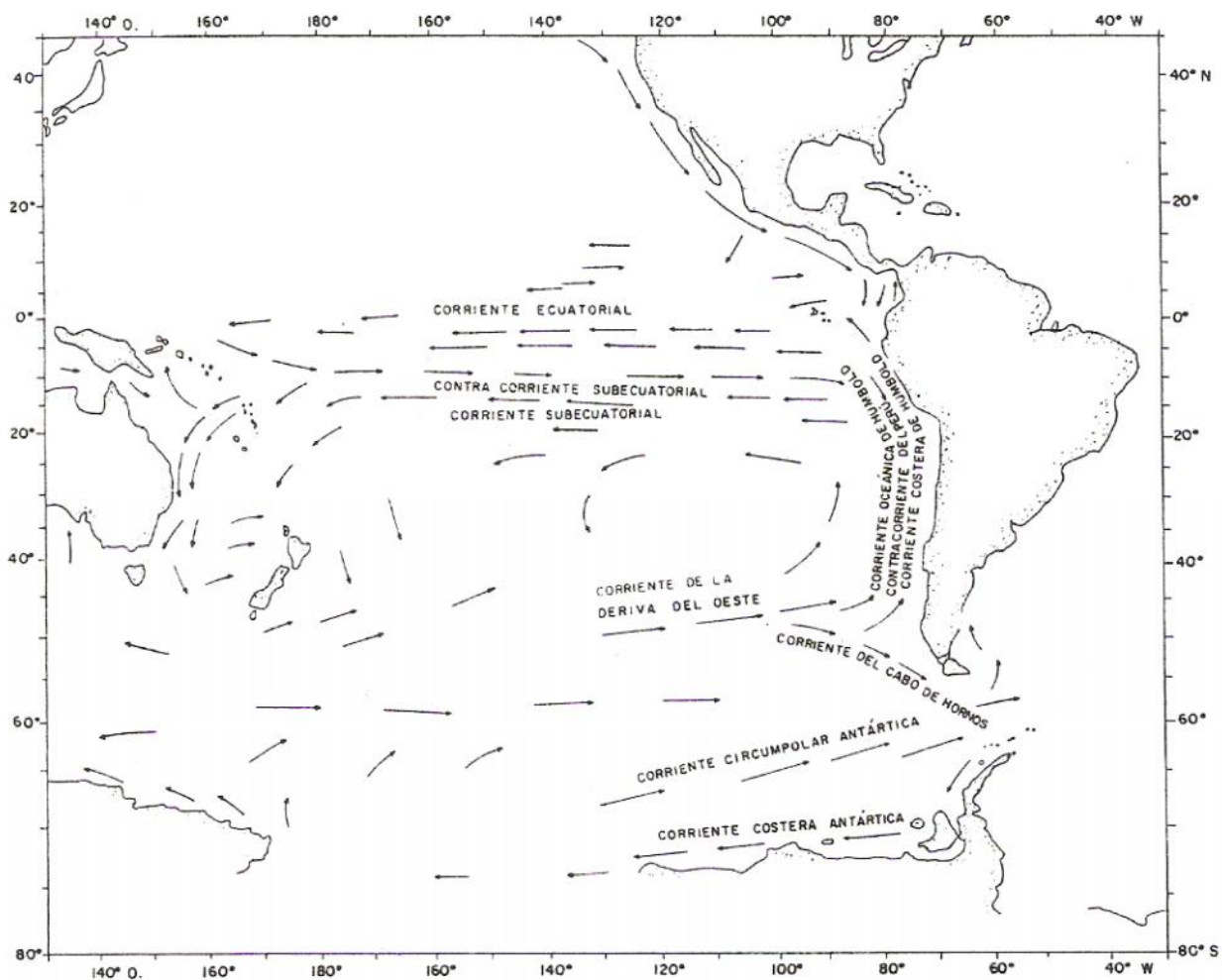
Fig. 43.—Sistema general de corrientes superficiales del océano Pacífico Sur.
