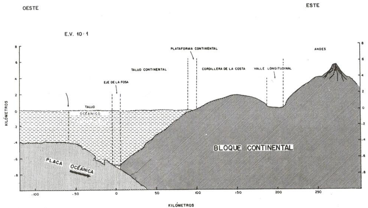
Fig. 4.—Corte frente al Chile central. El margen continental y la placa Oceánica que penetra por debajo del bloque continental.
