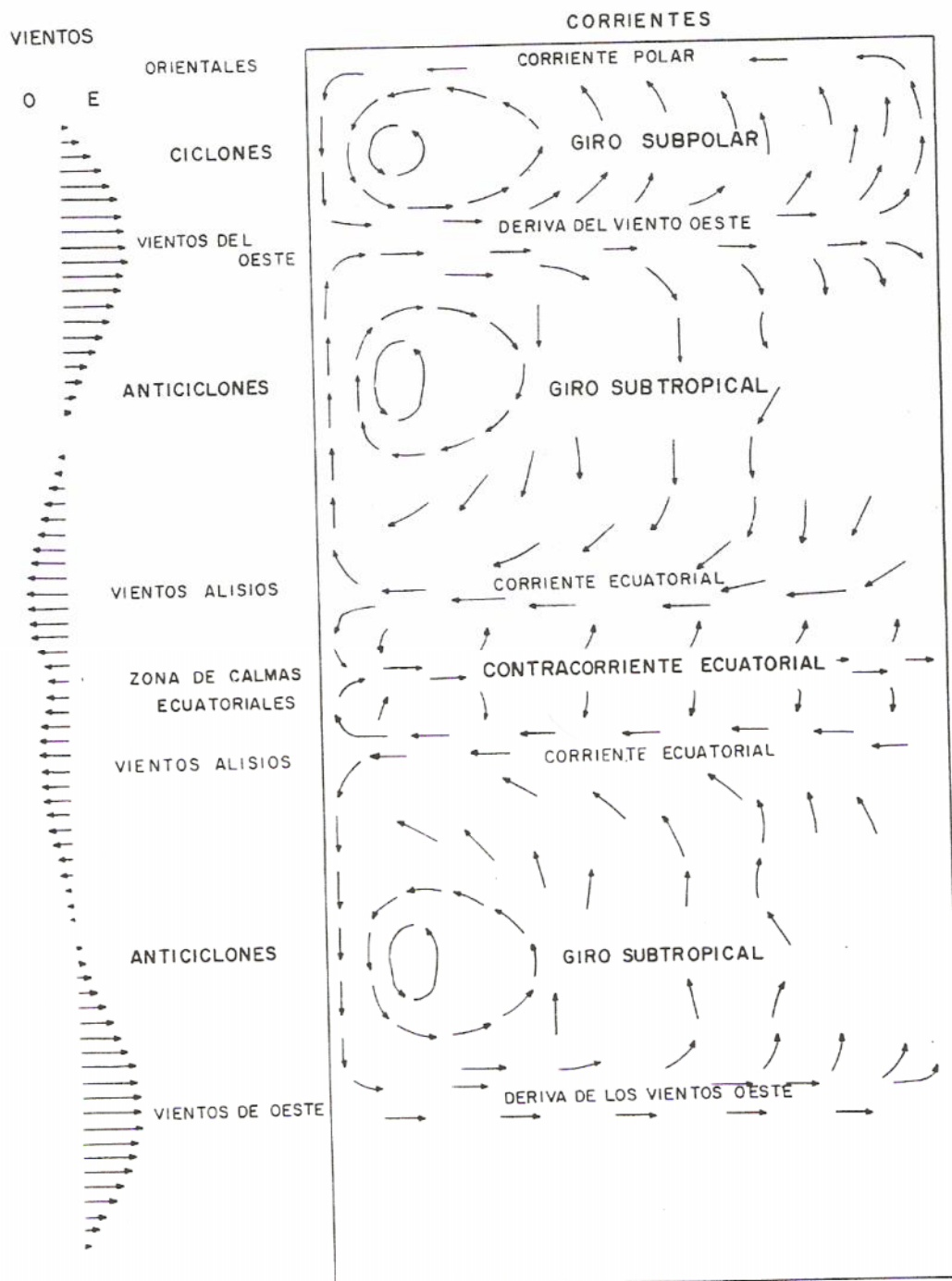
Fig. 42.—Diagrama de la circulación en un océano idealizado sometido sólo a la acción de los vientos.
