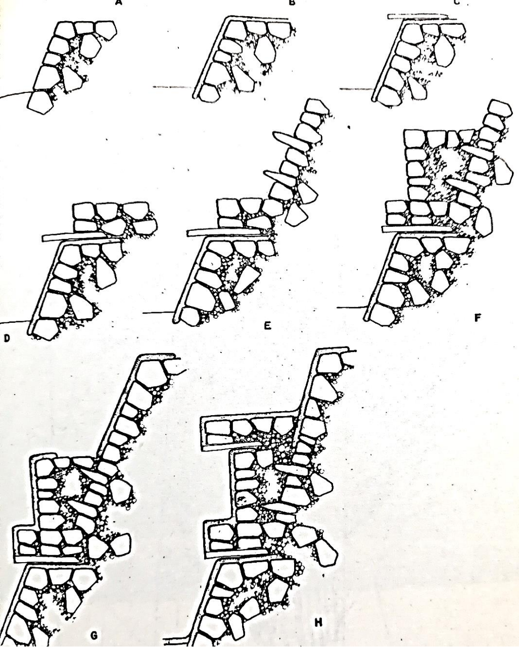
DIFERENTES FASES DE LA CONSTRUCCIÓN DE UN TALUD TABLERO TEOTIHUACANO. Marquina 1964. En Silva, O. (1997) Prehistoria de América. Ed Universitaria. Santiago. P.87
